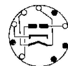
EZ80
