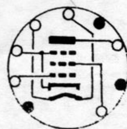
EL84
