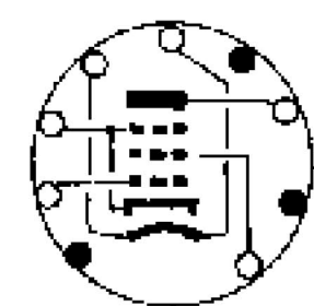
EL84
