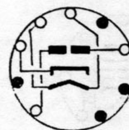
EZ80
