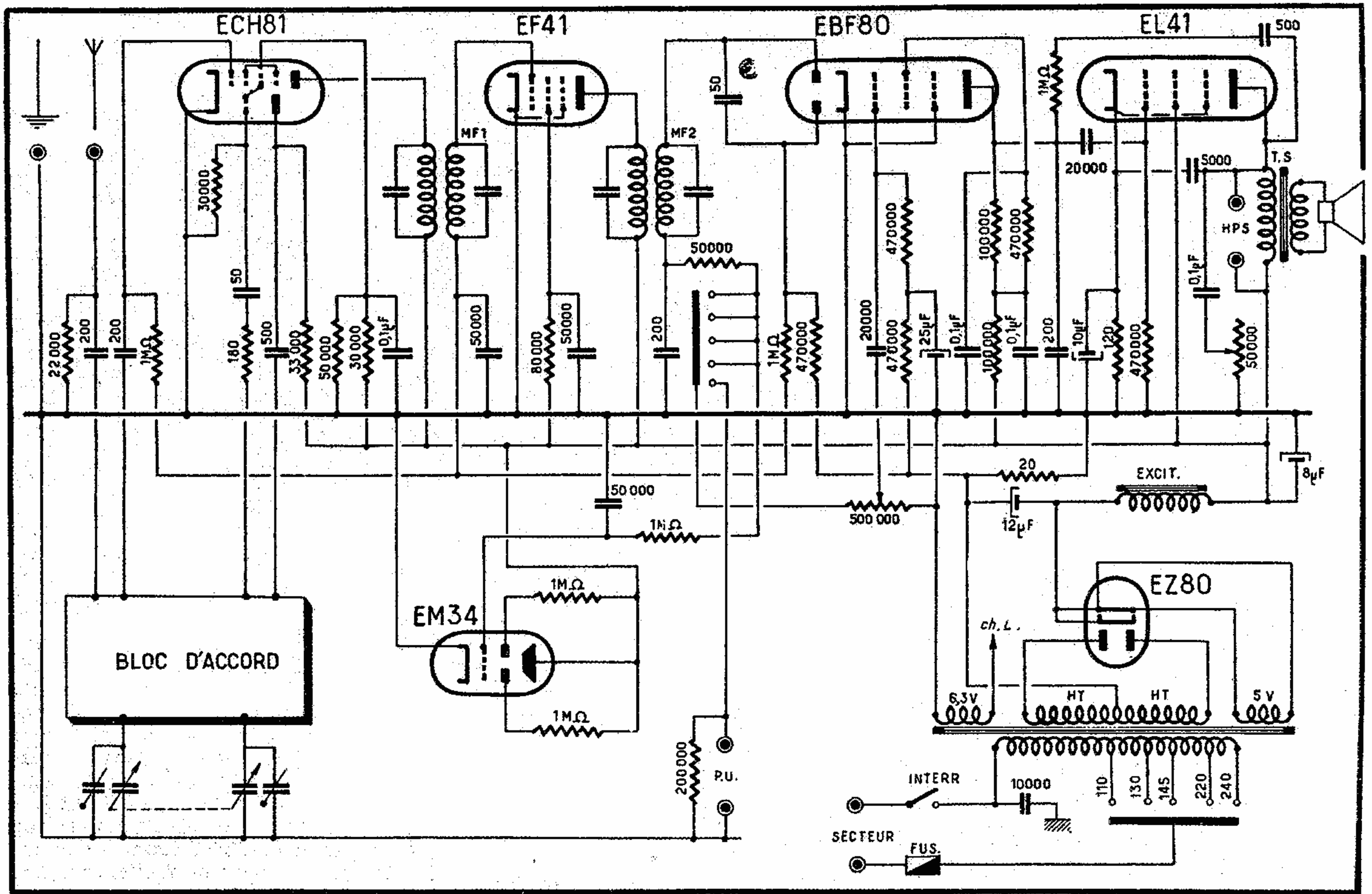
SCHÉMA DE PRINCIPE DU "COMPACT RADIO-PHONO"
