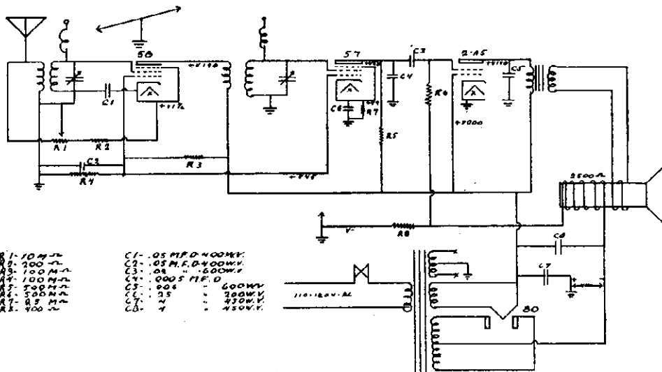
4 Tube T.R.F. 1934-1935
