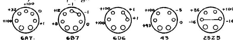
CHASSIS DAS. BOTTOM VIEW.
