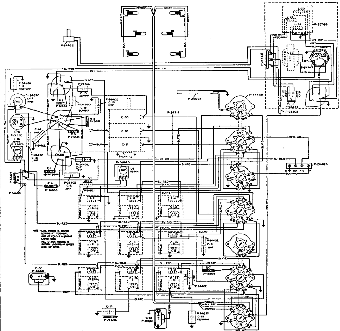
Fig. 3. Wiring Diagram.
