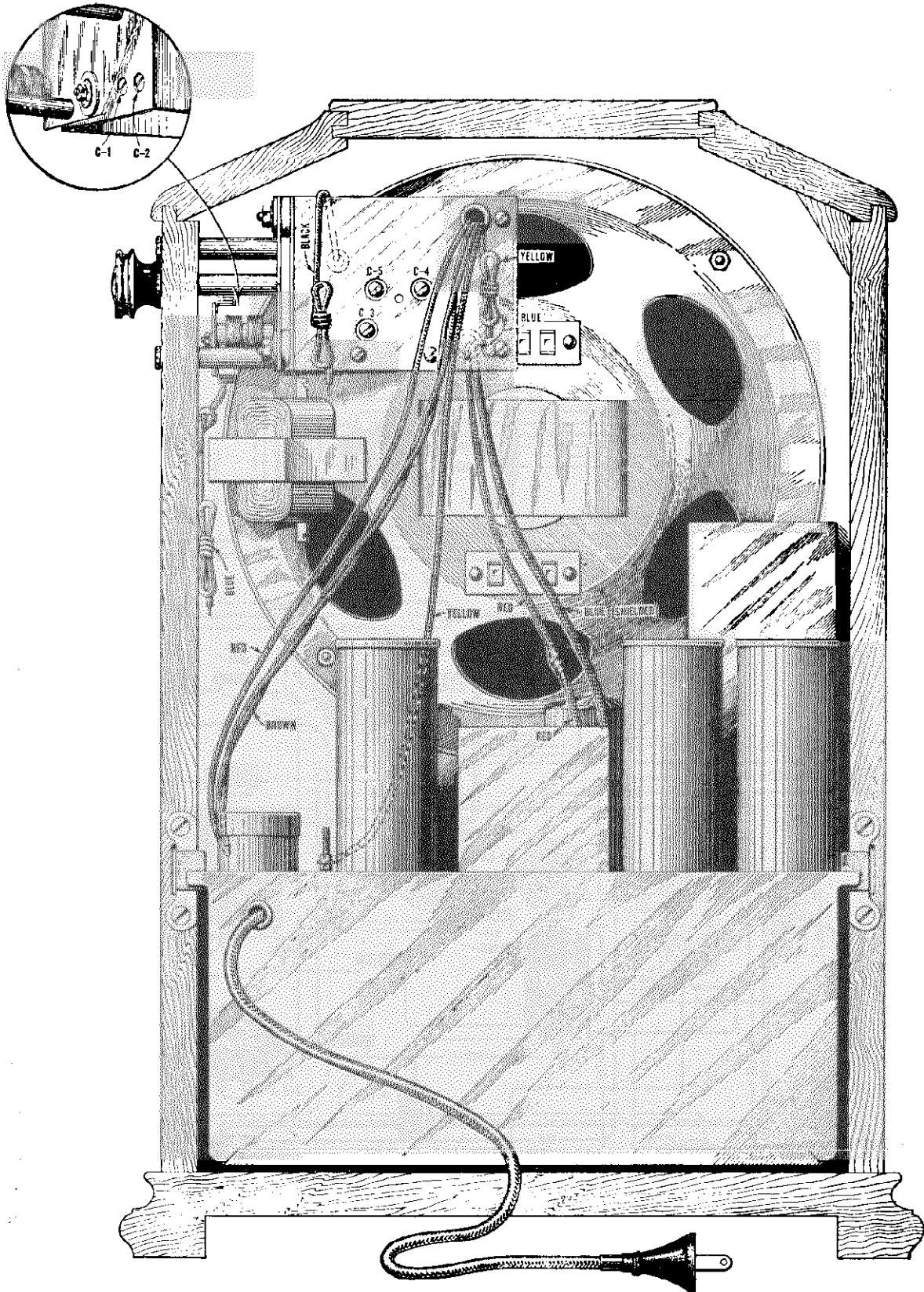
Figure 6—R-24-A Assembly Wiring
