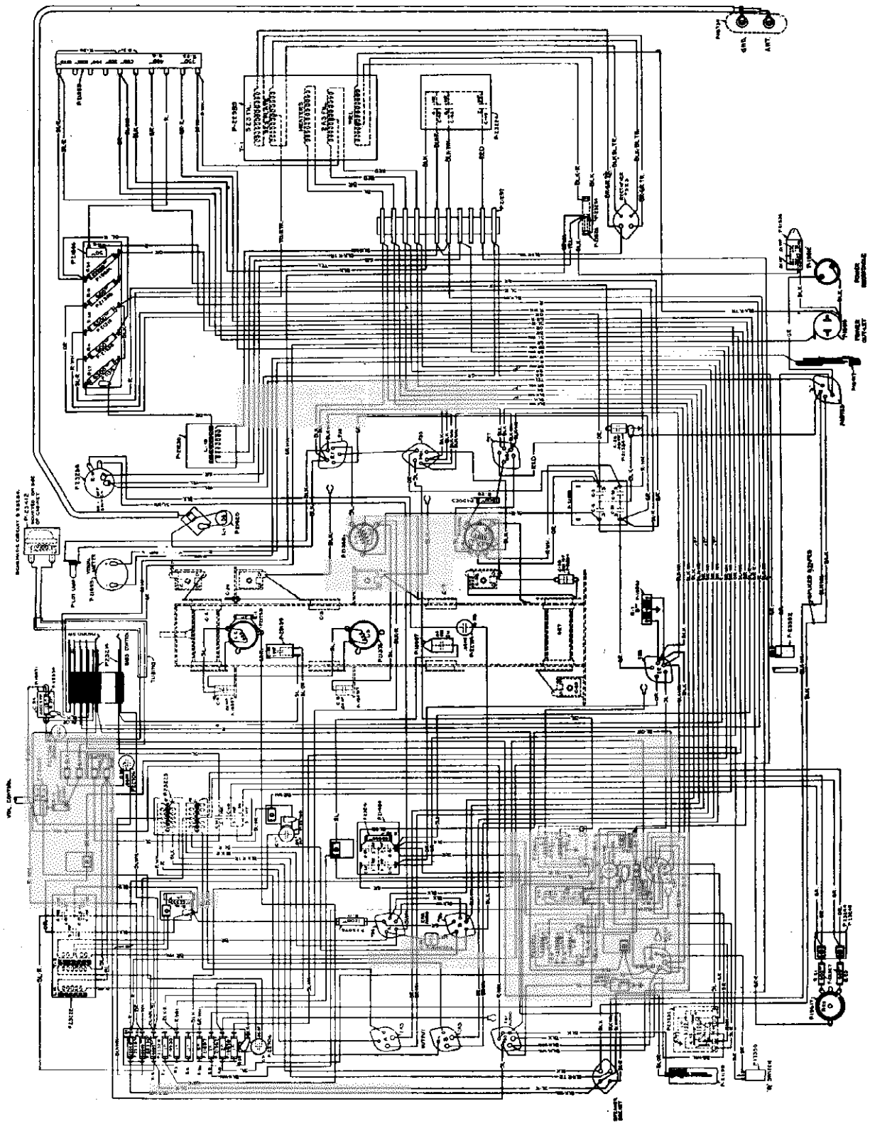
Fig. 1. Wiring Diagram.
