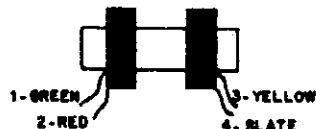
R-8039 LF. INPUT TRANSF.
