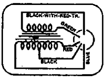
INPUT A. F. TRANSFORMER ASSEMBLY
