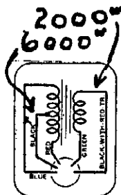
ONE A. F. INPUT TRANSFORMER
