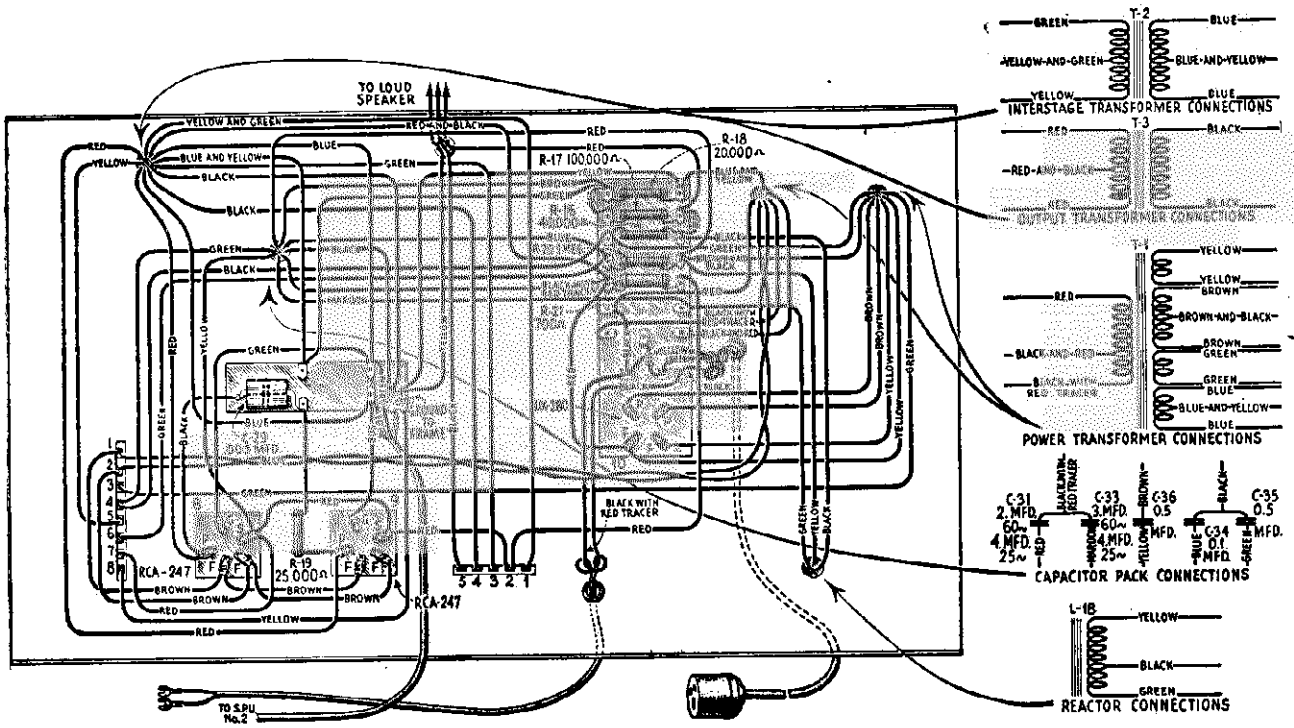
S. P. U. No. 1 wiring
