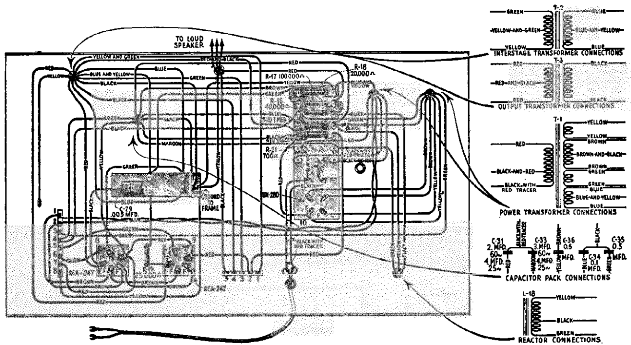
S. P. U. No. 2 wiring
