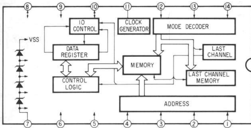
IC703 CX761A
