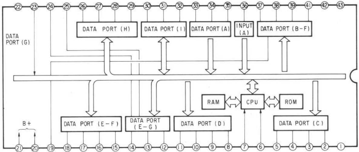
IC701 JPD553C
