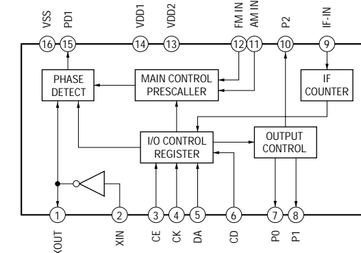
IC50 BU2614FS
