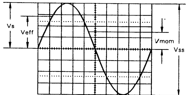
Spannungswerte an einer Sinuskurve
