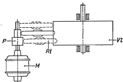
Fig. 30. Système d'entraînement de la bande pour trois vitesses de défilement. P = poulie à trois diamètres. Rt = galet intermédiaire en caoutchouc. VI = volant.
