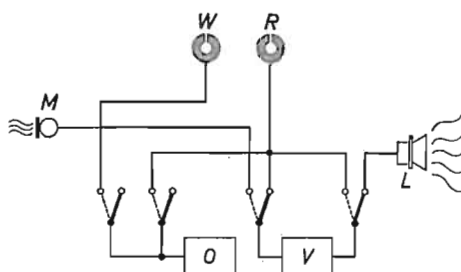
Fig. 28. Représentation schématique du circuit électronique dans un magnétophone simple.
