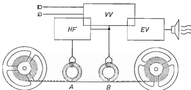
Fig. 27. Fonctions combinées dans un magnétophone.
