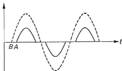
Fig. 22. Aimantation de la bande par suite du courant. A = lorsqu'il n'y a aucune pr magn tisation. B = avec pr magn tisation.
