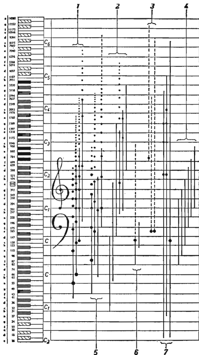
Fig. 2. Spectre de fréquence des instruments et des voix.
