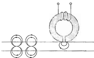
Fig. 23. Concentration des lignes de force   travers la t te lors de la reproduction.
