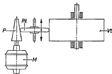
Fig. 31. Système d'entraînement de la bande à galet intermédiaire réglable et poulie conique. P = poulie conique. Rt = galet intermédiaire réglable. VI = volant.
