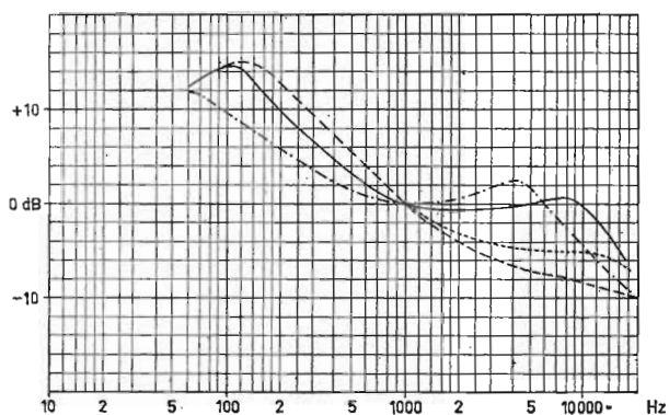
Fig. 26. Caractéristiques de fréquence d'un magnétophone 4 vitesses.
