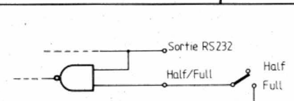
Fig. 2. — Commutation half/full du-plex du terminal vidéo de décembre.
