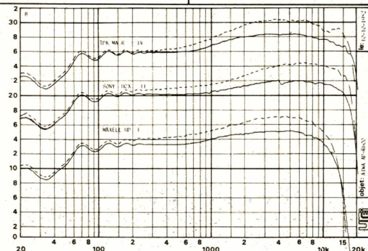
Courbes de réponse en fréquences ; en pointillé, nous lisons dans l'autre sens ce qui vient d'être enregistré après avoir retourné la cassette.
