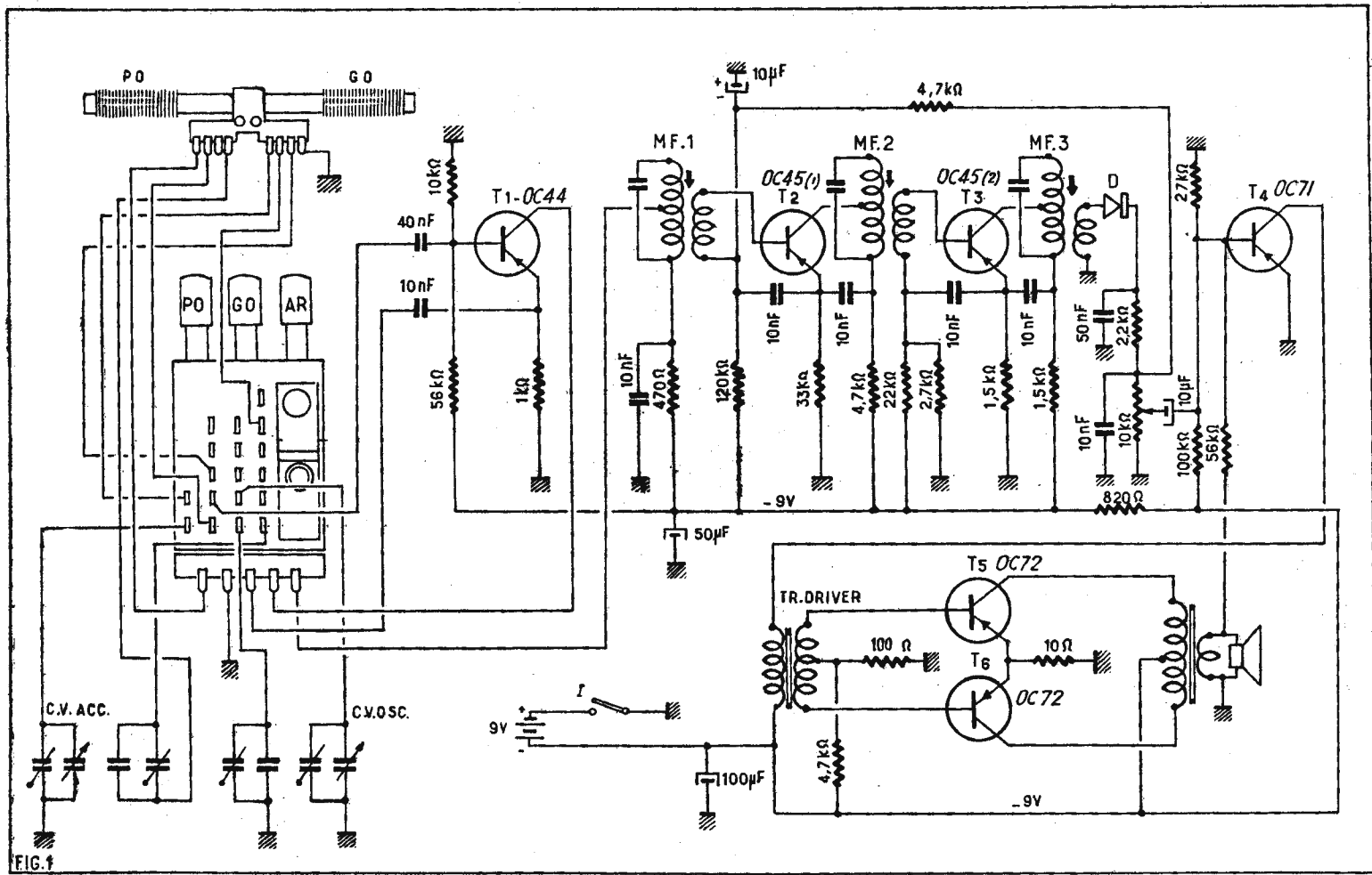
RÉCEPTEUR MINIATURE A 6 TRANSISTORS
