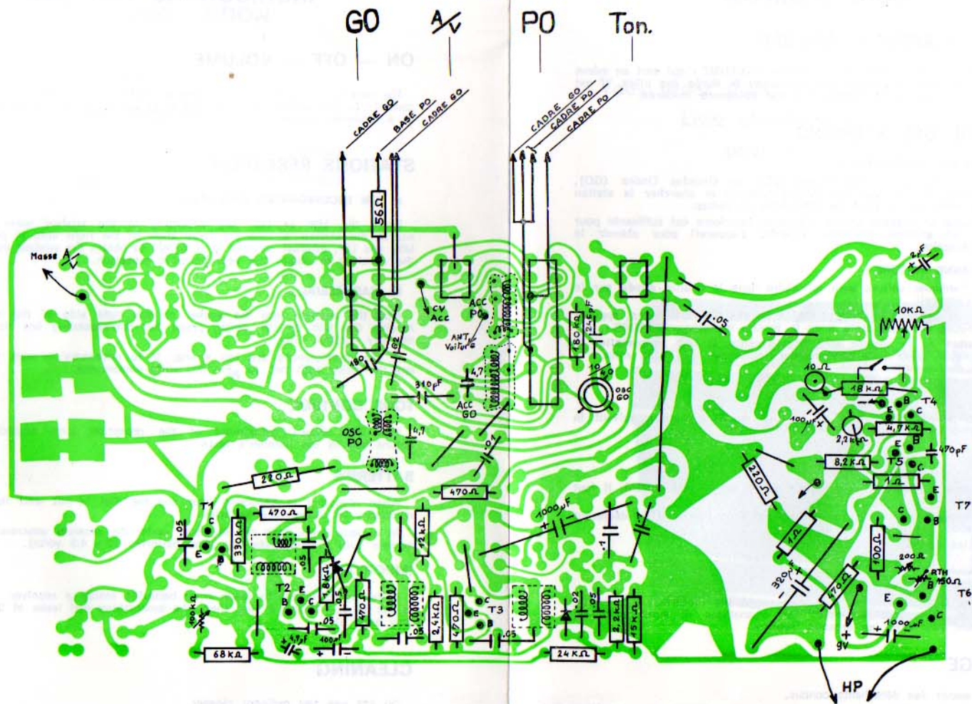
CIRCUIT IMPRIME VU COTE CUIVRE
