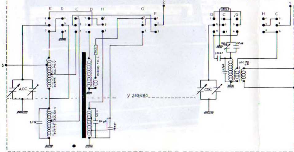
SCHEMA DE PRINCIPE
