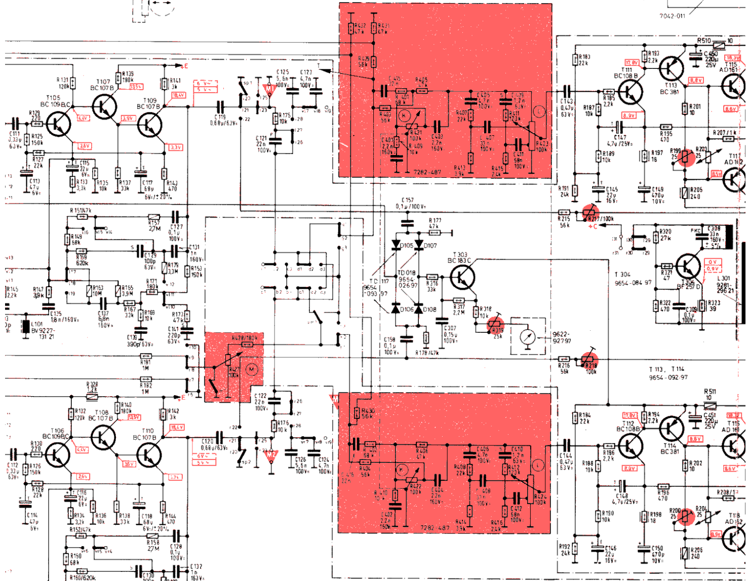
gezeichnete Schalterstellung Halt, Wiedergabe SWITCH POSITION IS/IS SHOWN STOP, PLAYBACK DESSINEE POSITION DU COMMUTATEUR ARRET, LECTURE COMMUTATORE RAPPRESENTATO IN POSIZIONE STOP, ASCOLTO
