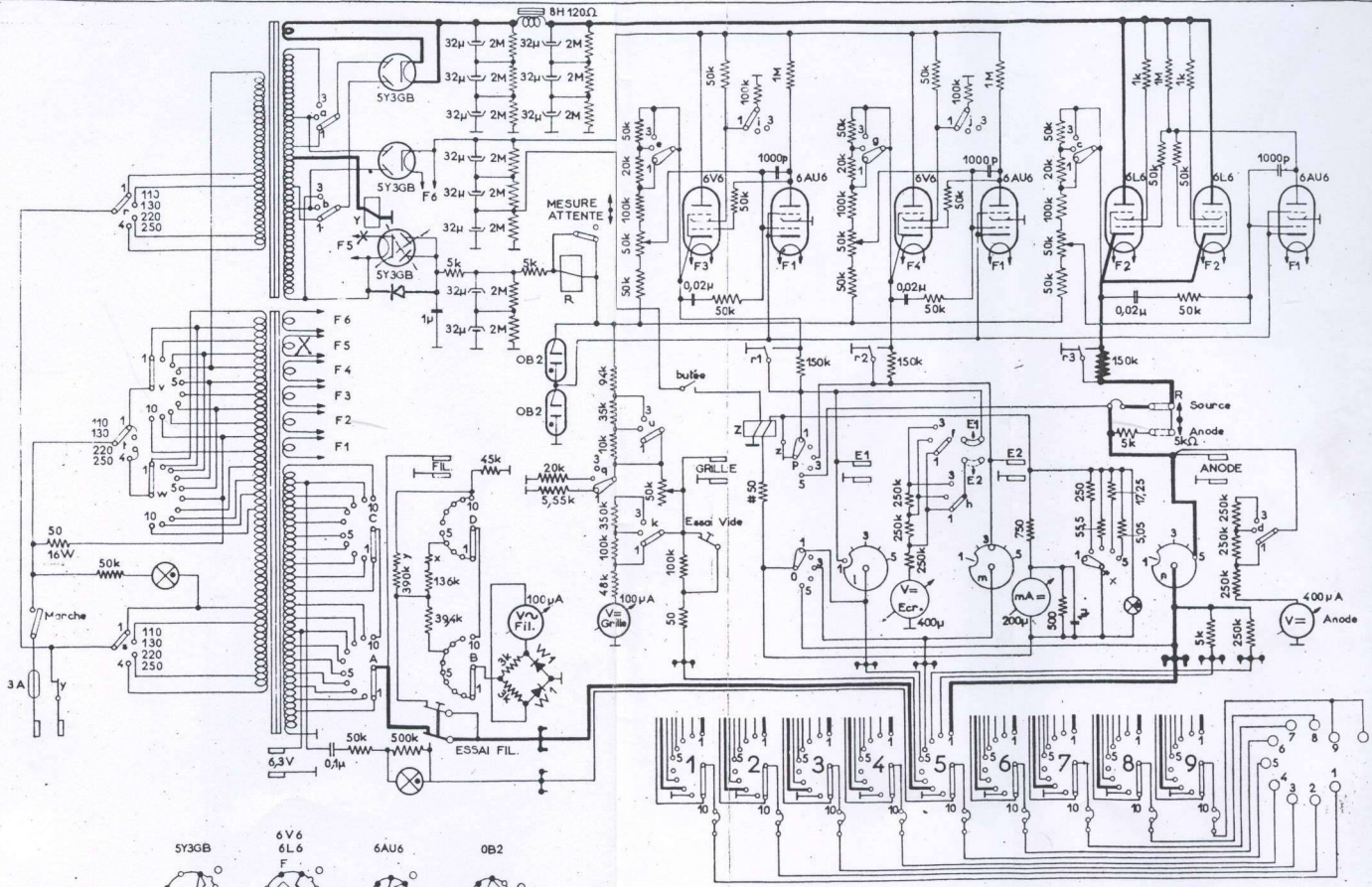
Schéma de principe TRU61.B
