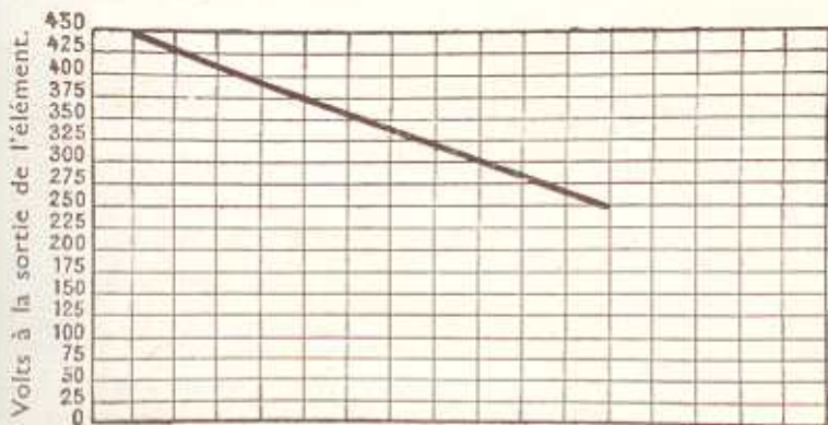
Élément HT 5 - 6 - 7
