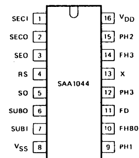
Fig. 2 Pinning diagram.
