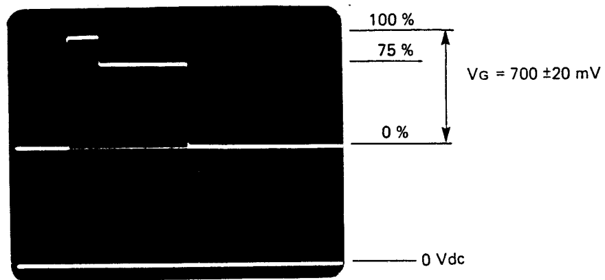
Fig. 35 Output 'GREEN'
