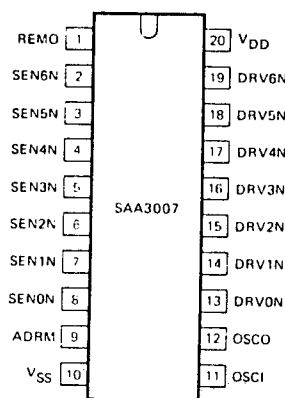
Fig. 2 Pinning diagram.
