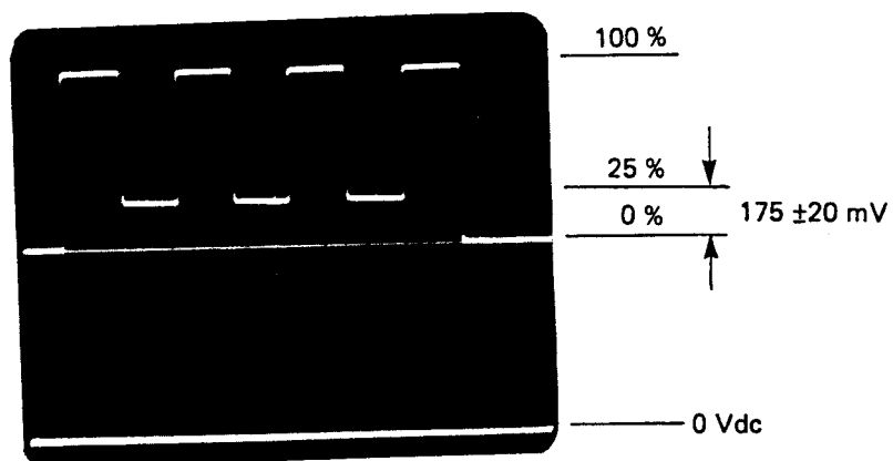
Fig. 48 Output 'BLUE'
