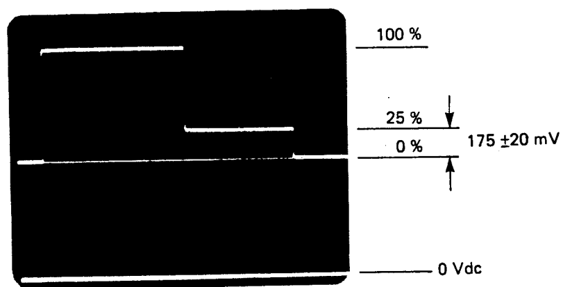
Fig. 47 Output 'GREEN'
