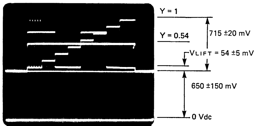
Fig. 37 Output 'RED'
