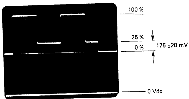
Fig. 46 Output 'RED'
