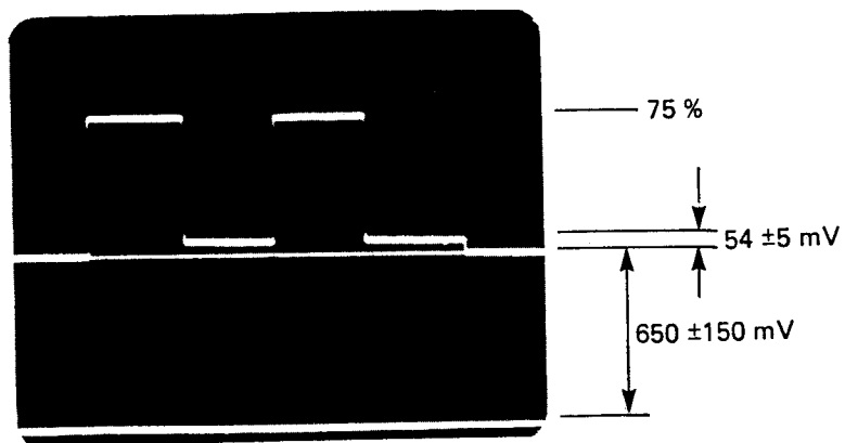
Fig. 40 Output 'RED'
