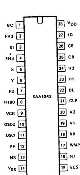
Fig. 2 Pinning diagram.
