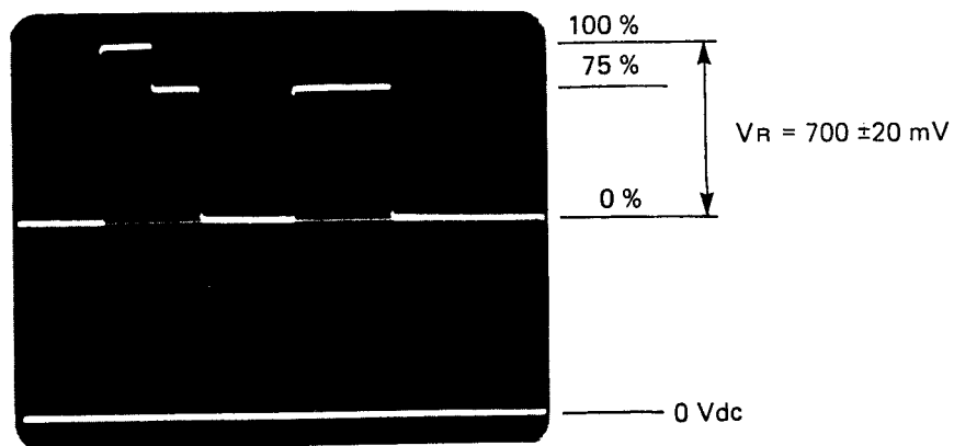
Fig. 34 Output 'RED'
