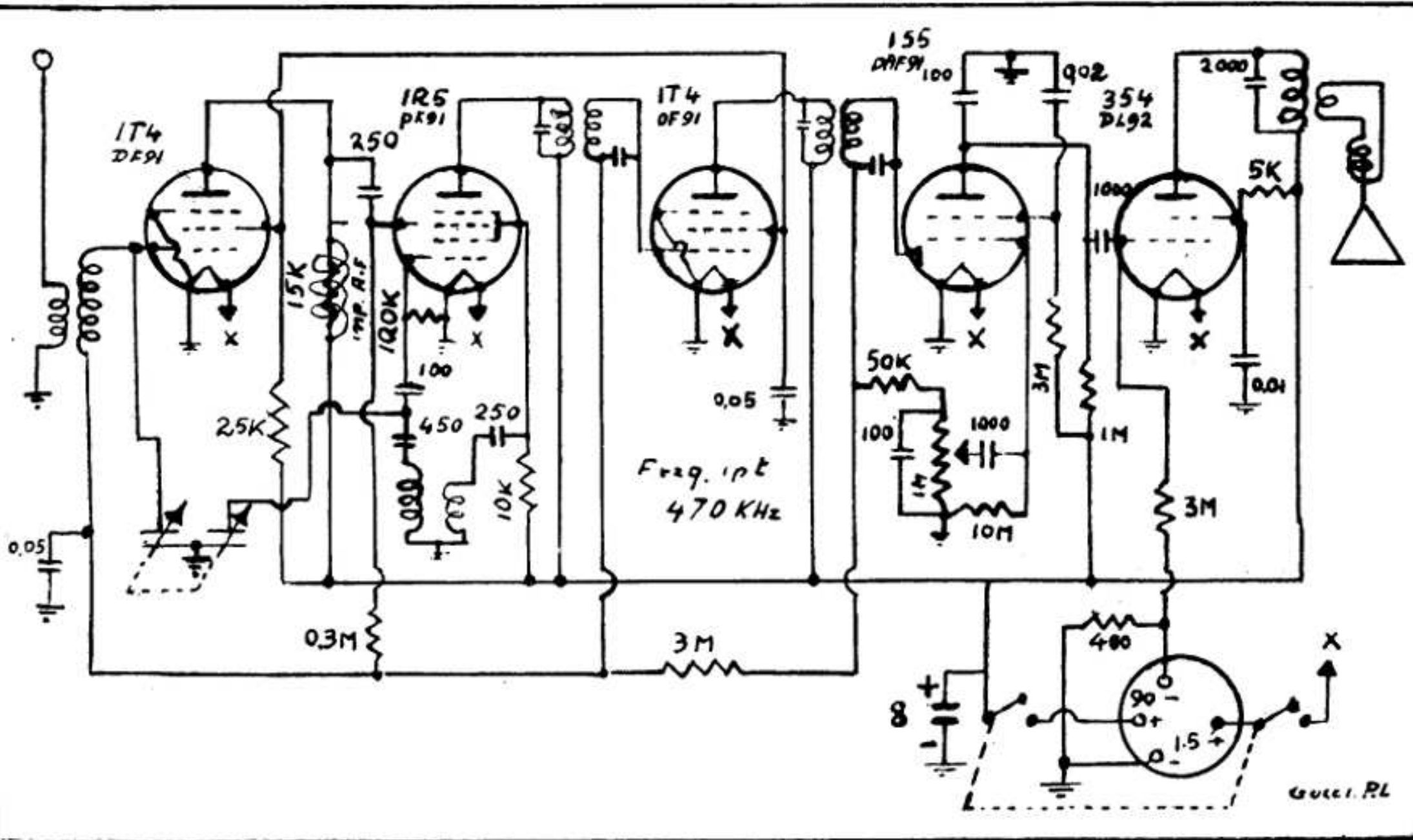
ALTAR - Mod. MOTO-SCOOTER. Apparecchio alimentato a pile, adatto per moto-scooter. Gamma onde medie da 180 a 510 metri. Media frequenza 467 kc/s.
