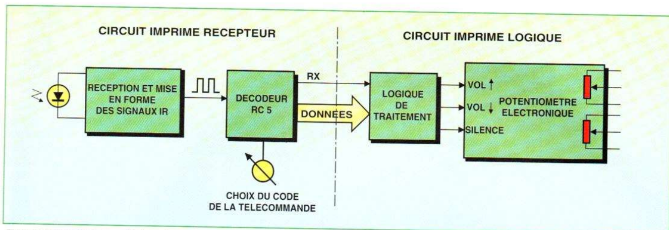
Figure 1 : Synoptique complet de notre montage.
