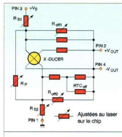
Figure 6 - Constitution interne du MPX 2200 AP
