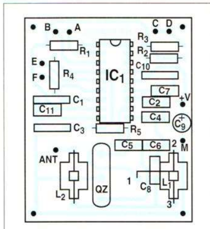
Figure 3 : Implantation des composants.
