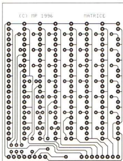
Figure 10 - Circuit imprimé, de la matrice de LED, côté cuivre, échelle 1.
