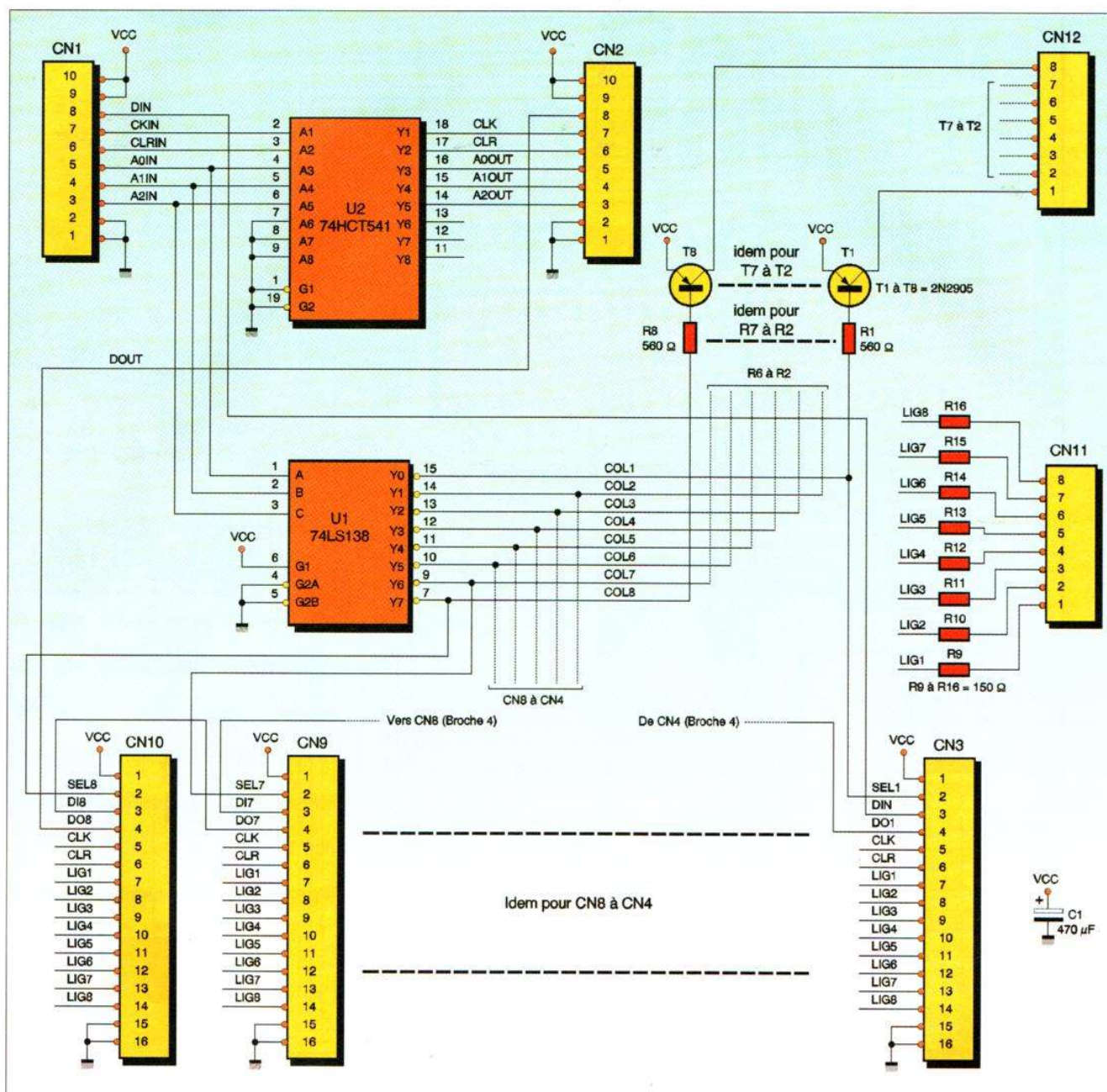
Figure 3 - Schéma de principe d'une carte de base
