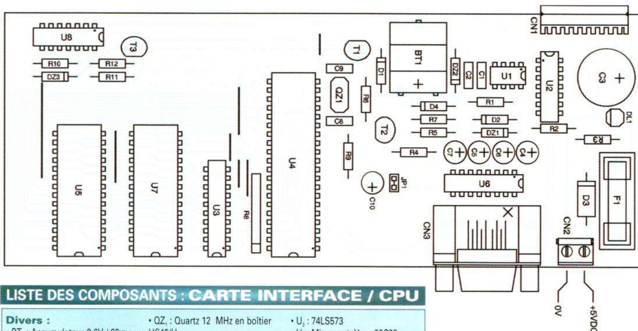
Figure 7 - Implantation des composants de la carte interface.
