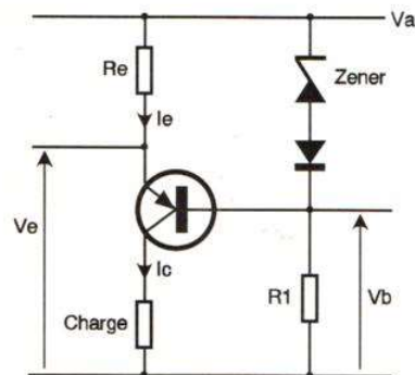
... et sa version nettement plus stable.
