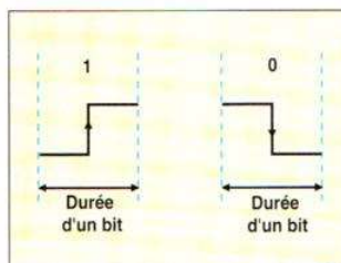
Figure 2 : Principe du codage biphase utilisé en RC5.
