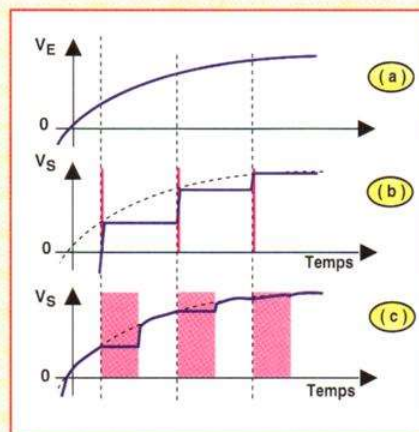
Figure 5 - Pour les signaux de haute fréquence, tels que les signaux vidéo, on utilise souvent une variante de ce circuit dénommée "Track & Hold" ("suiveur-bloqueur"). La fréquence d'échantillonnage étant très élevée (plusieurs MHz), il n'est pas nécessaire de disposer d'une capacité CH importante (la décharge entre deux échantillonnages consécutifs est négligeable). Si l'on bloque le signal entre les impulsions - figure 4(b) -, le rattrapage à effectuer à chaque impulsion est important. Or il est simplement nécessaire de le bloquer, c'est à dire le maintenir constant, pendant la conversion. Le reste du temps, le signal peut être appliqué à la sortie. La faible valeur du condensateur (47 pF par exemple, contre 1 000 pF et au-delà pour un circuit plus classique) lui permet d'être connecté en permanence en dehors des périodes de blocage. Par conséquent, il est plus facile de faire l'acquisition précise de la valeur du signal, puisque la sortie le "suit" en permanence, sauf lors des blocages.
