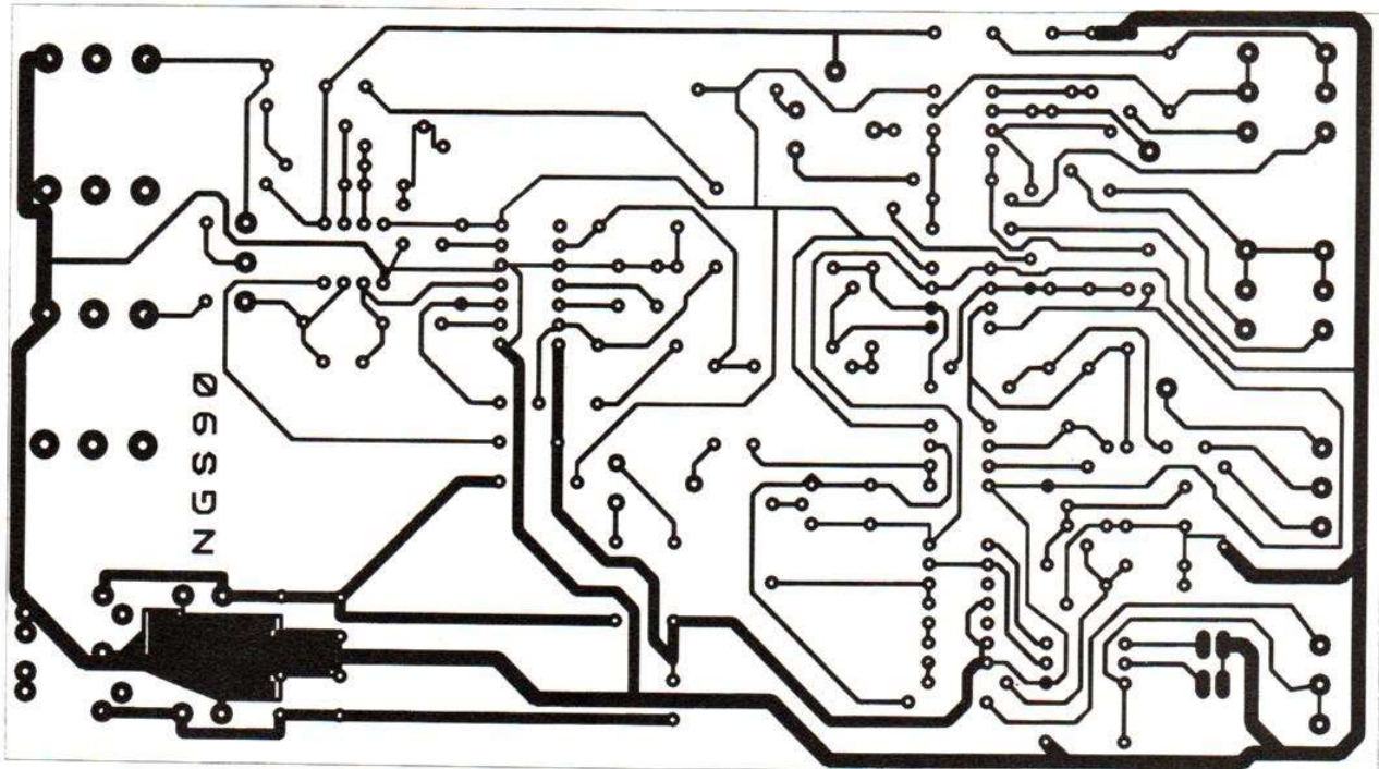
Figure 1 - Circuit imprimé du noise Gate Sélectif, échelle 1.
