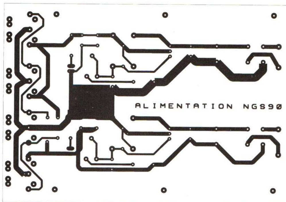
Figure 3 - Circuit imprimé de l'alimentation, échelle 1.
