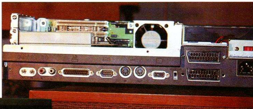
Façade arrière, avec les différents connecteurs.
