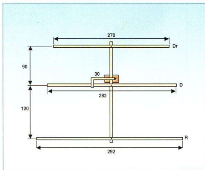
Figure 1 : Antenne 50 MHz à 3 éléments : dimensions en cm.
