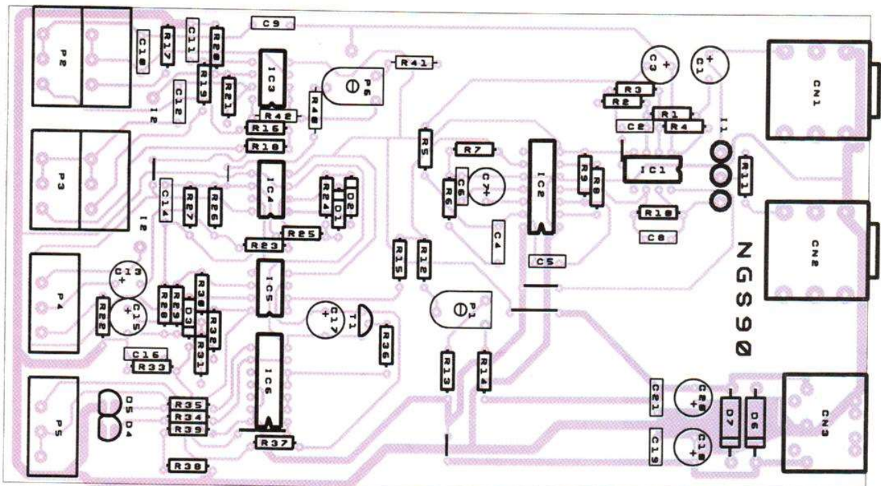
Figure 2 - Implantation des composants sur le circuit imprimé.
