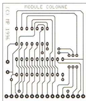
Figure 12 - Circuit imprimé, du module colonne, côté cuivre, échelle 1.
