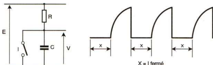
Le principe de production de dents de scie est fort simple ...
