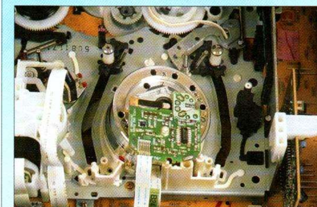
Installé au-dessus du tambour, un amplificateur de tête audio M.F. attaque un transformateur spécialisé. Le tambour est monté sur une semelle de matière plastique qui sert aussi de butée aux doigts de guidage de la bande, montés eux-aussi sur une matière plastique..
