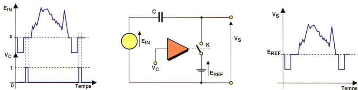
Figure 8 Le circuit de "clamp" actif est une intéressante variante du précédent, dans laquelle la diode D est remplacée par un commutateur électronique K actionné par une commande extérieure V_C . La commande est une impulsion qui encadre la zone du signal que l'on désire "aligner" sur la tension de référence, par exemple une fraction du palier arrière de suppression ligne.
