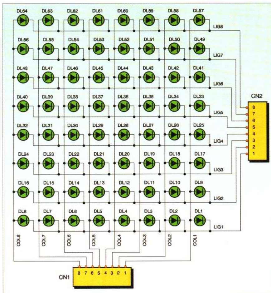
Figure 4 - Schéma de principe d'une matrice à LED.
