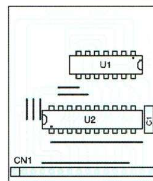
Figure 13 - Implantation des composants du module colonne.
