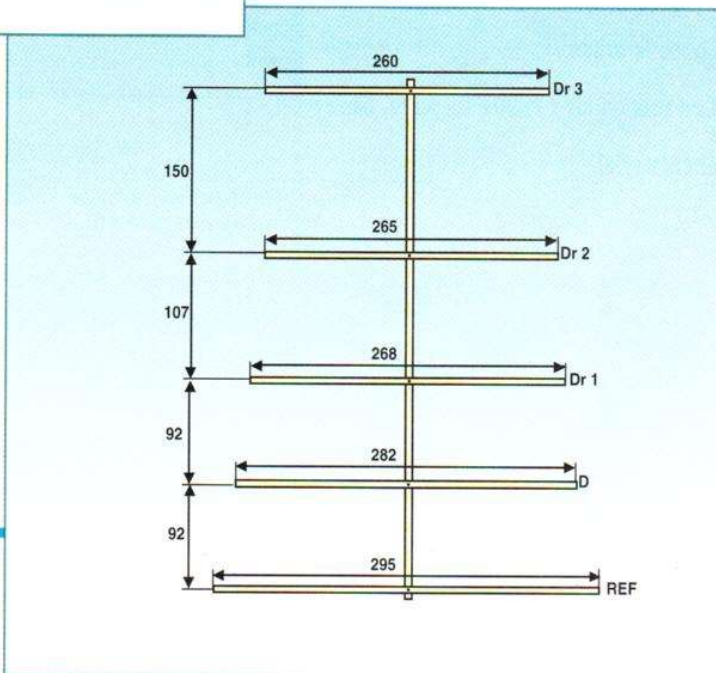
Figure 7 : Antenne cinq éléments 50 MHz (dimen- sion en cm).
