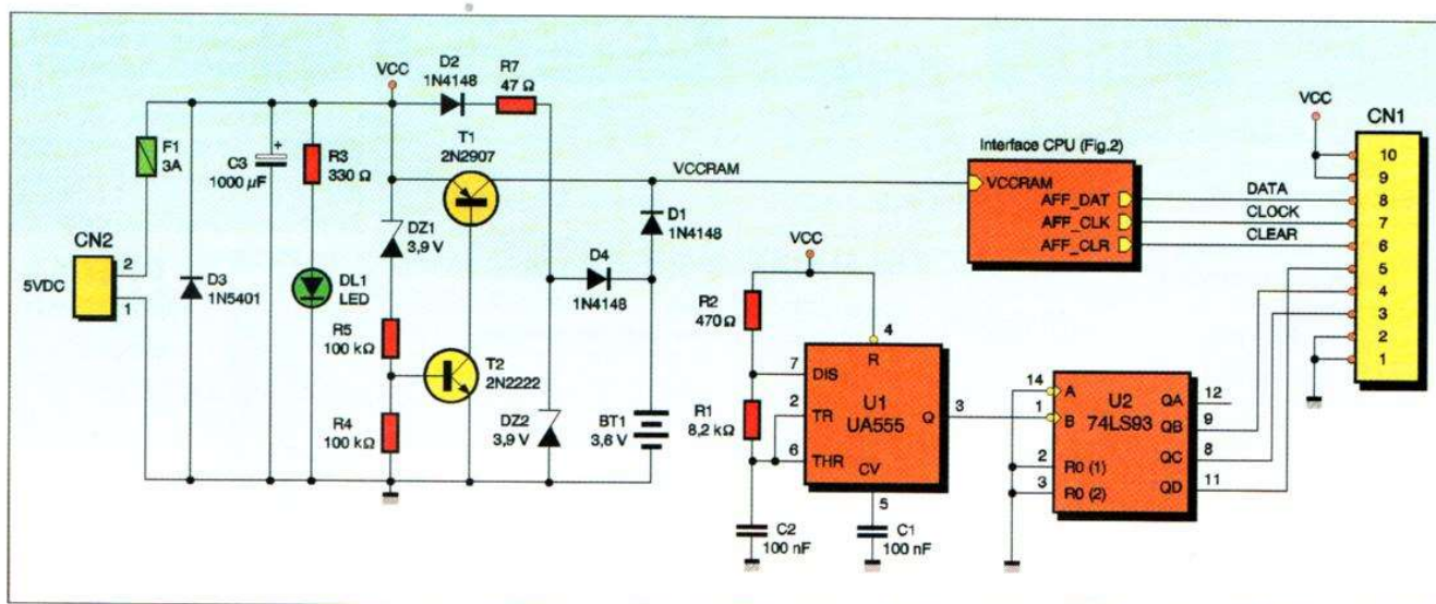
Figure 1 - Schéma de principe de l'alimentation sauvegardée et de l'horloge auxiliaire.
