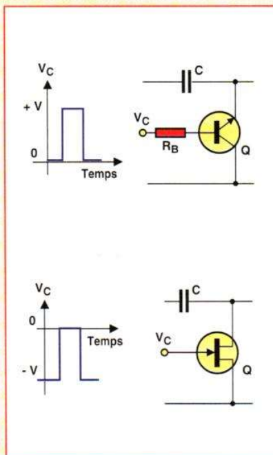
Figure 9 - Le commutateur peut-être: un pont de diodes, un transistor bipolaire-figure 9(a), un transistor à effet de champ-figure 9(b) -, ou bien un commutateur analogique intégré à base de technologie JFET (transistors à effet de champ à jonction), MOS ou CMOS. L'avantage certain du montage actif est qu'il permet de "clamper" à n'importe quel endroit du signal: fond des impulsions de synchro, palier de suppression, etc., et que, si l'interrupteur choisi laisse passer le courant dans les deux sens (ce qui est le cas des commutateurs analogiques intégrés), il permet de compenser les variations du signal d'entrée dans les deux sens.
