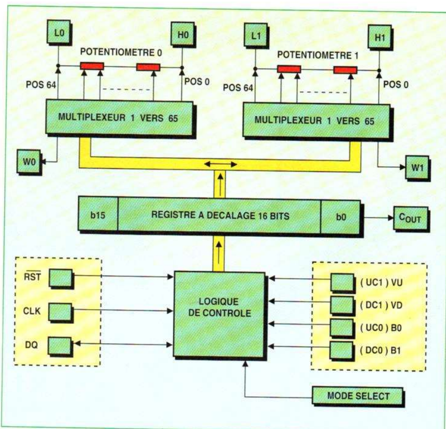
Figure 2 : Synoptique interne du potentiomètre électronique DS 1802.
