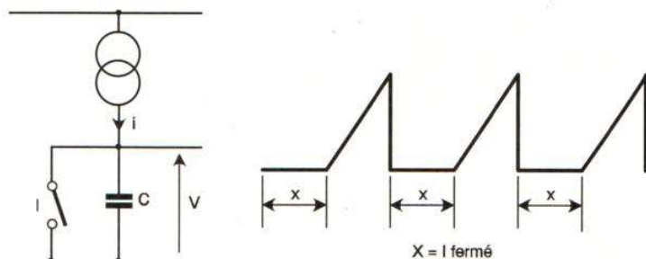
Pour produire des dents de scie linéaires, il faut un générateur à courant constant.
