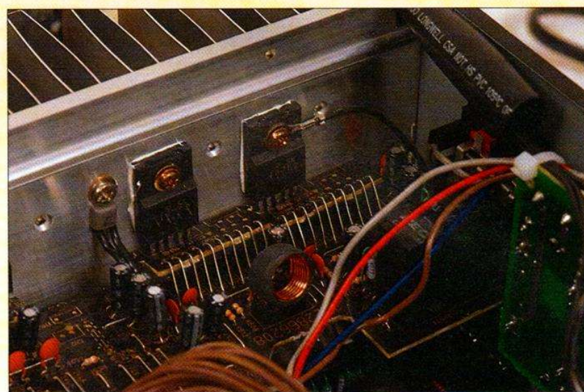
Des circuits intégrés sont chargés de l'amplification des canaux arrière. Le constructeur prévoit une double implantation, le circuit imprimé est un morceau de la plaque de base sur laquelle ont été installés des straps par une machine automatique.
