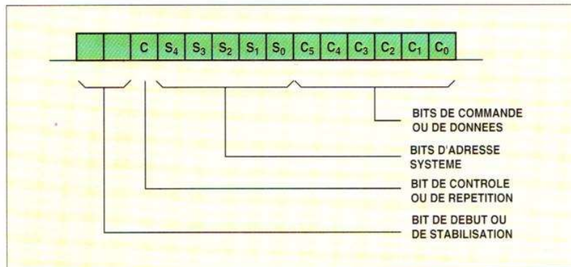
Figure 1 : Structure d'un message en code RC5.
