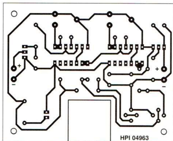
Figure 2 : Circuit imprimé, vu côté cuivre, échelle 1
