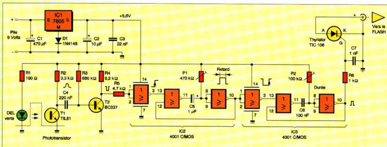
Figure 1 : Schéma de notre montage
