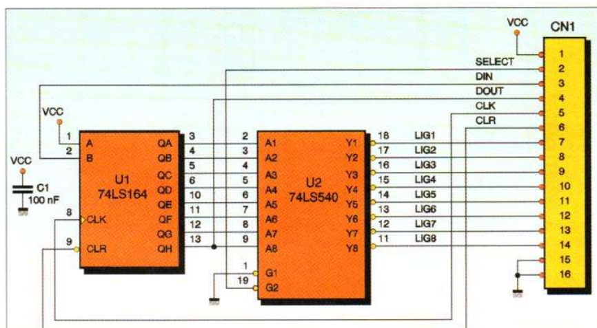
Figure 4 - Schéma de principe d'une matrice à LED.
