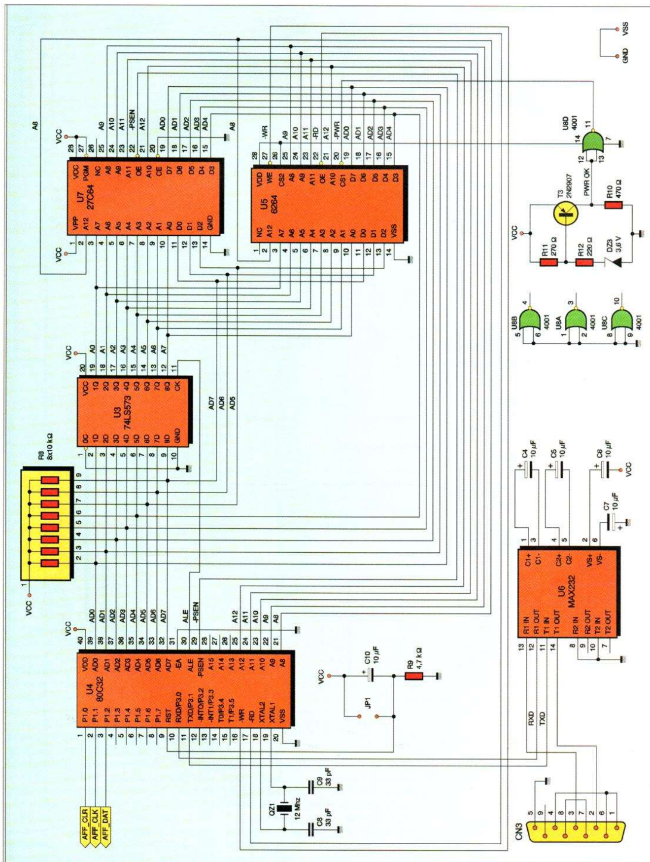
Figure 2 - Schéma de principe de la carte interface
