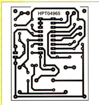
Figure 2 : Circuit imprimé, vu côté cuivre, échelle 1
