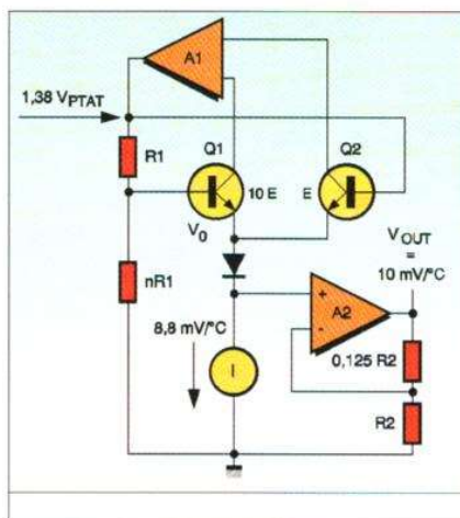
Figure 5 - Schéma interne du capteur de température.
