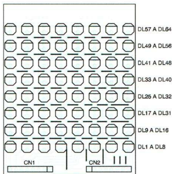
Figure 11 - Implantation des composants de la matrice de LED.
