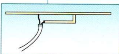
Figure 4 : Le gamma match
