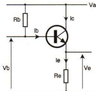
Les deux schémas classiques du collecteur commun
