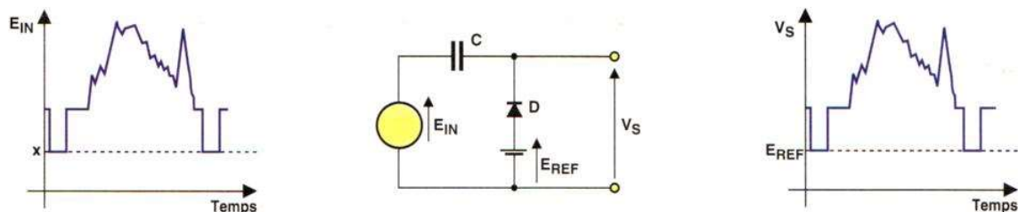
Figure 6 - Le circuit d'alignement passif met en œuvre un condensateur C et une diode D . Lorsque le signal d'entrée E_{IN} est inférieur à la tension E_{REF} , la diode D devient conductrice et charge le condensateur C . Dès que la tension E_{IN} redevient supérieure à E_{REF} , la diode cesse de conduire, et le signal est transmis intégralement. La capacité C joue donc le rôle de mémoire, et reste chargée à une valeur de tension égale à la différence entre E et la valeur de crête la plus négative de E_{IN} . Avantage: circuit simple à fonctionnement automatique. Inconvénients: l'énergie nécessaire à la charge de C est prélevée sur la
