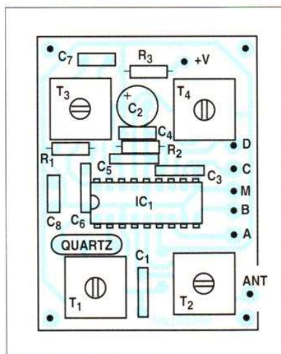
Figure 3 : Implantation des composants.
