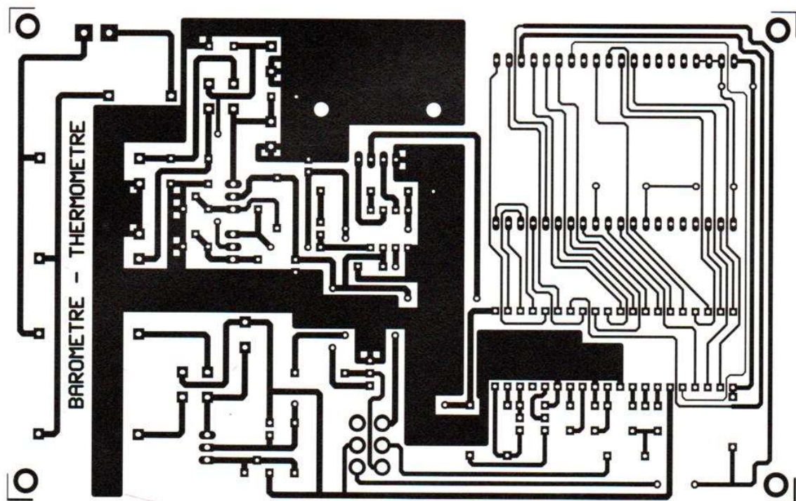
Figure 7 - Circuit imprimé de notre thermomètre - baromètre digital.
