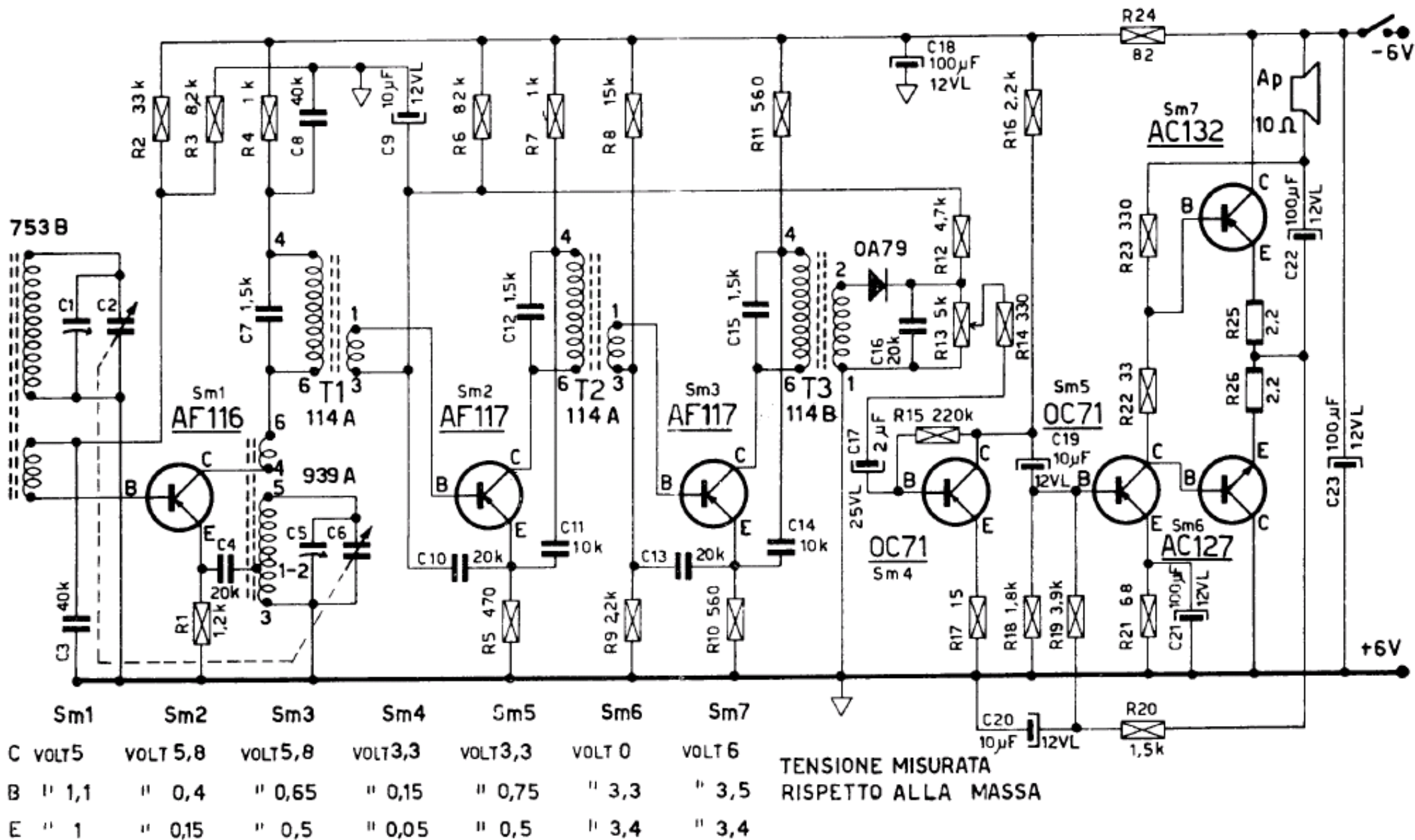
Schema elettrico del radiorecettore ALLOCCIO BACCHINI mod. 2014
