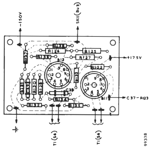
Fig. 43. Gedrukte-bedradingsplaat van unit F
