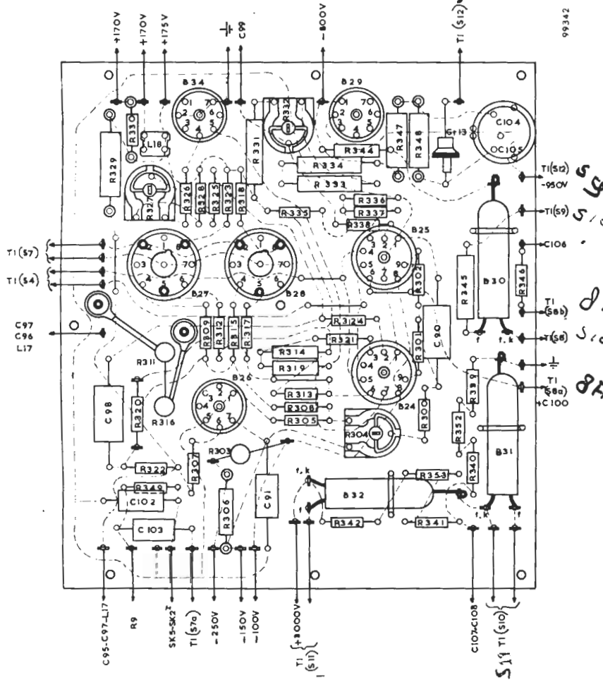
Fig. 47. Gedrukte-bedradingsplaat van unit K
