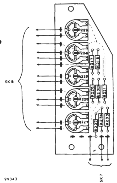
Fig. 48. Gedrukte-bedradingsplaat van unit L
