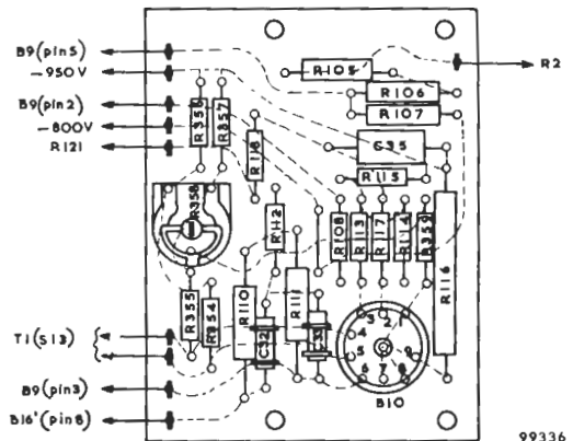
Fig. 41. Gedrukte-bedradingsplaat van unit D
