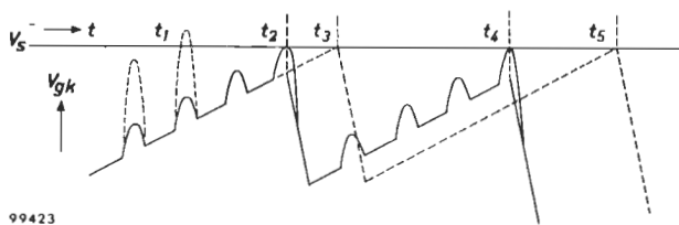
Fig. 9. Spanningsvorm tussen rooster en katode van B_{20}
