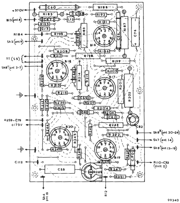
Fig. 45. Gedrukte-bedradingsplaat van unit H
