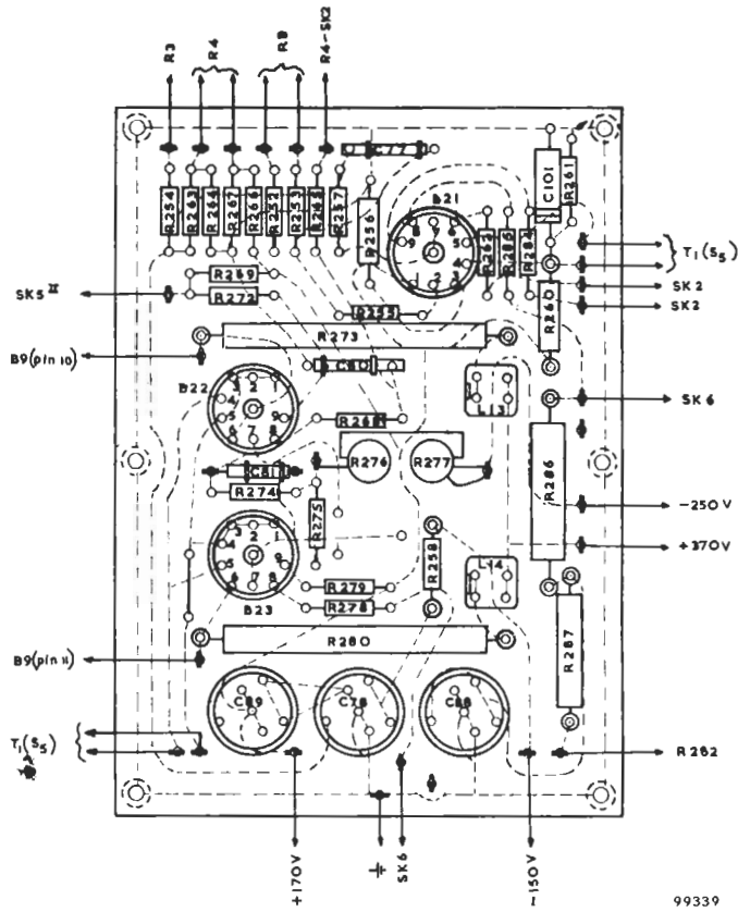
Fig. 44. Gedrukte-bedradingsplaat van unit G
