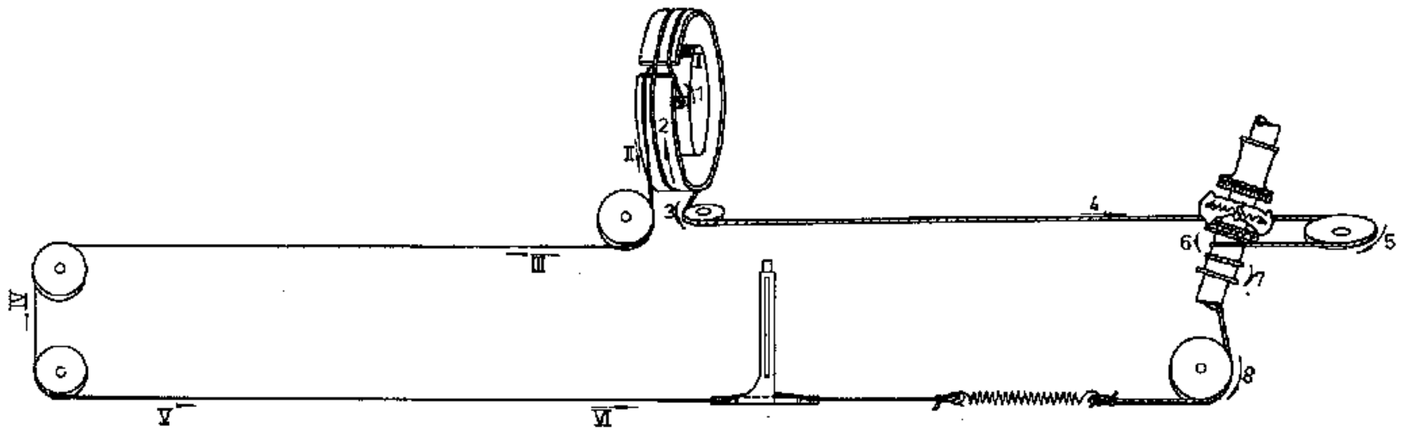
FM-Skalenseil-Verlauf für Antrieb 422 WR / 434 WR
