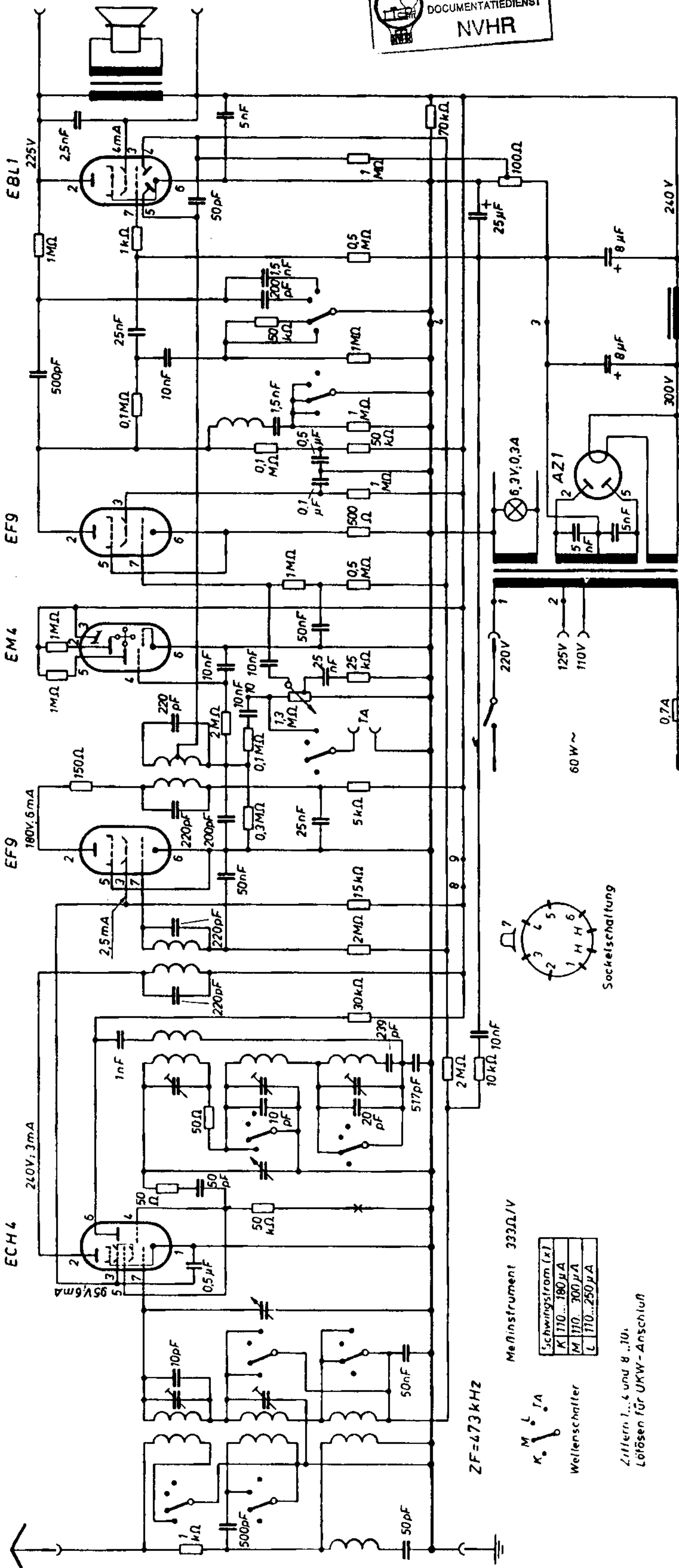
AEG 1469 WK Konzert-Super
