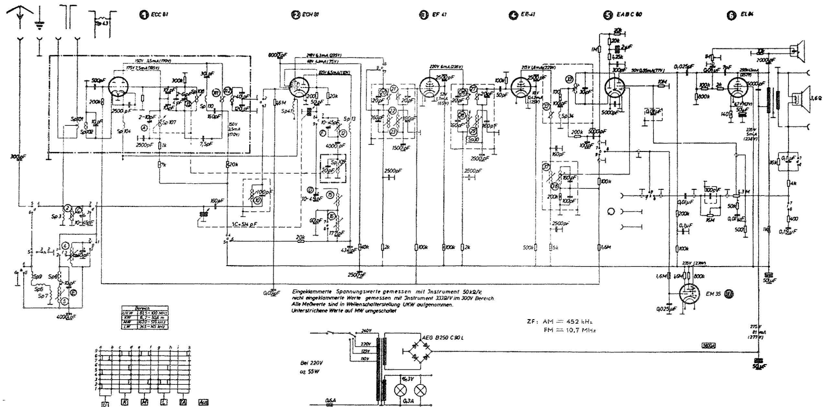
Prinzip-Schaltbild mit Strom-Spannungswerten des AEG Wechselstrom - Supers „AEG 2073 WU“
