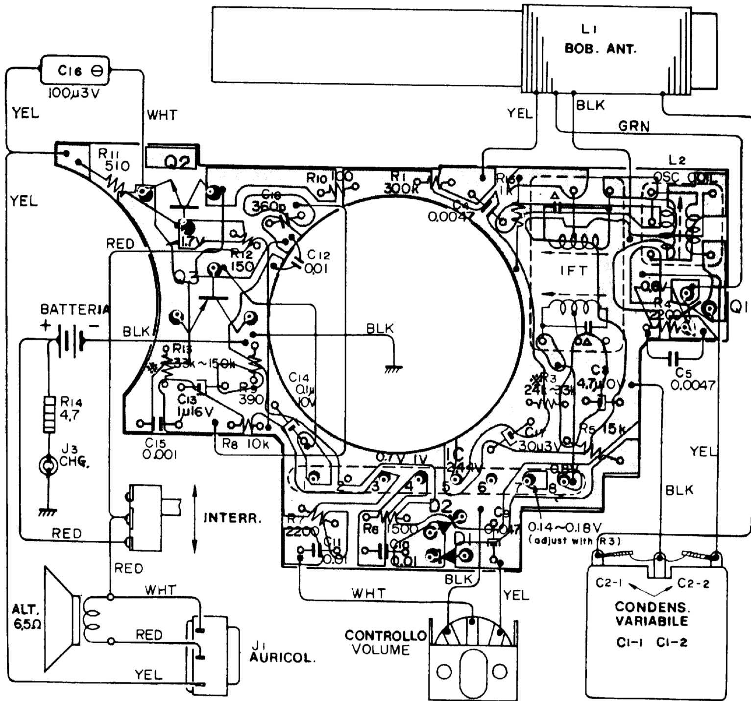
Fig. 8.25. - Circuito stampato e componenti.
