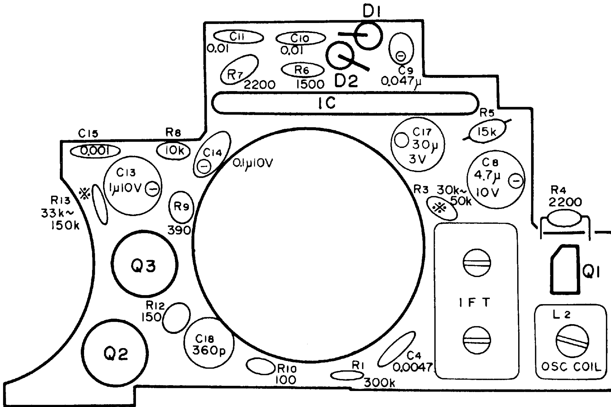
Fig. 8.23. - Pannellino e componenti.
