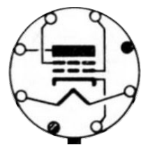
6L6G
