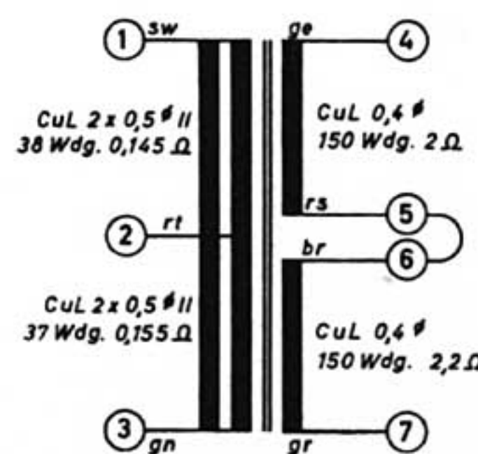
BV 9048-501 Ausgangstrafo Output Transformer Transfo de sortie
