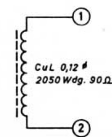
BV 9281-080 Sperrkreisspule Rejection Coil Bobine de réjection
