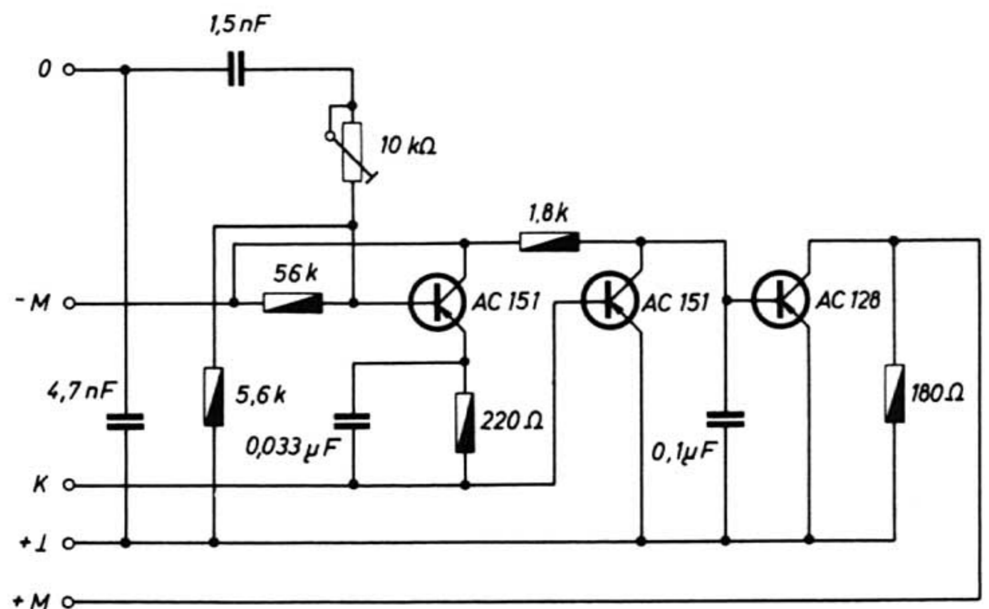
Schaltbild Motorplatte 7281-164
