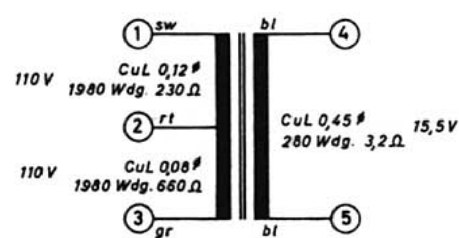
BV 9003-510 Netztrafo Mains Transformer Transfo secteur
