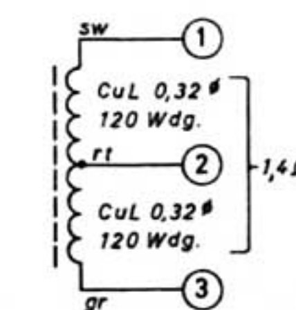
BV 9281-099 Saugkreisspule Absorption Coil Bobine d'absorption
