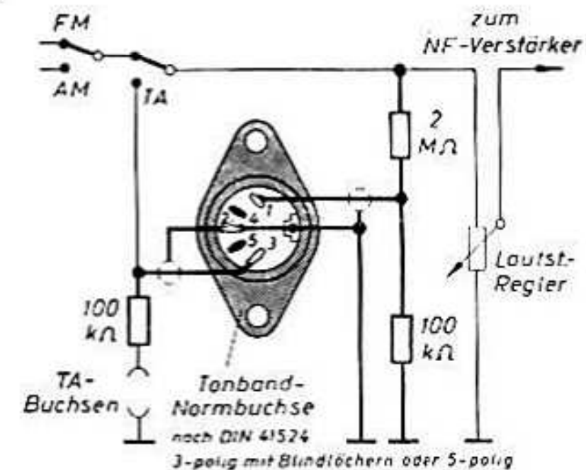
Abb. 2 Blick auf die Lötanschlüsse der Buchse
