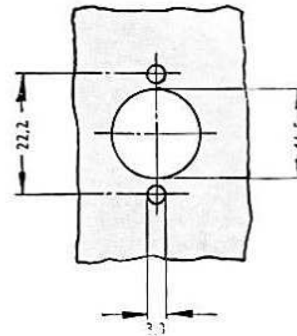
Abb. 1 Ausschnitt an Chassis-Rückseite Maße in mm
