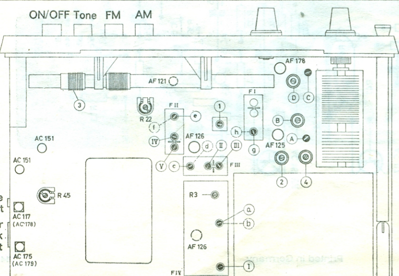
Abgleich-Lageplan ALIGNMENT SCHEME PLAN DE REGLAGE PIANO DI TARATURA
