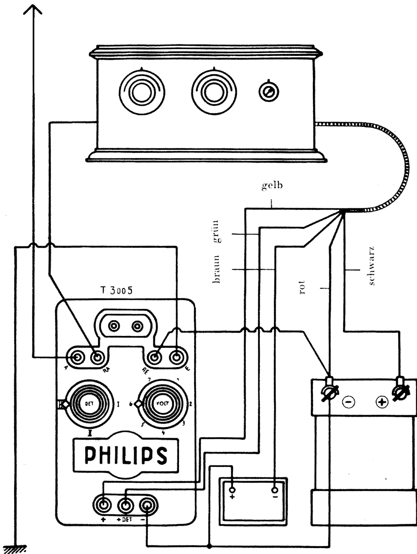
Anschluss des Philips-Volksempfängers an das Philips-Netzanschlussgerät T 3005 (Gleichstrom-Lichtnetz).
