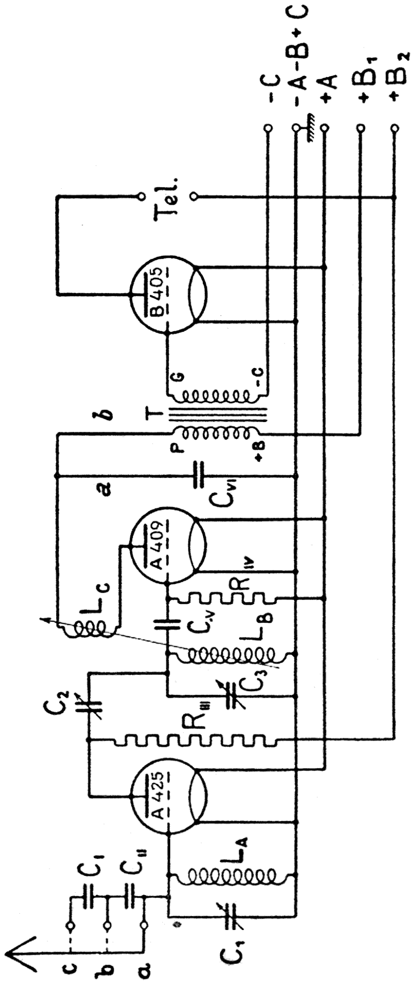
Das Schaltschema.
