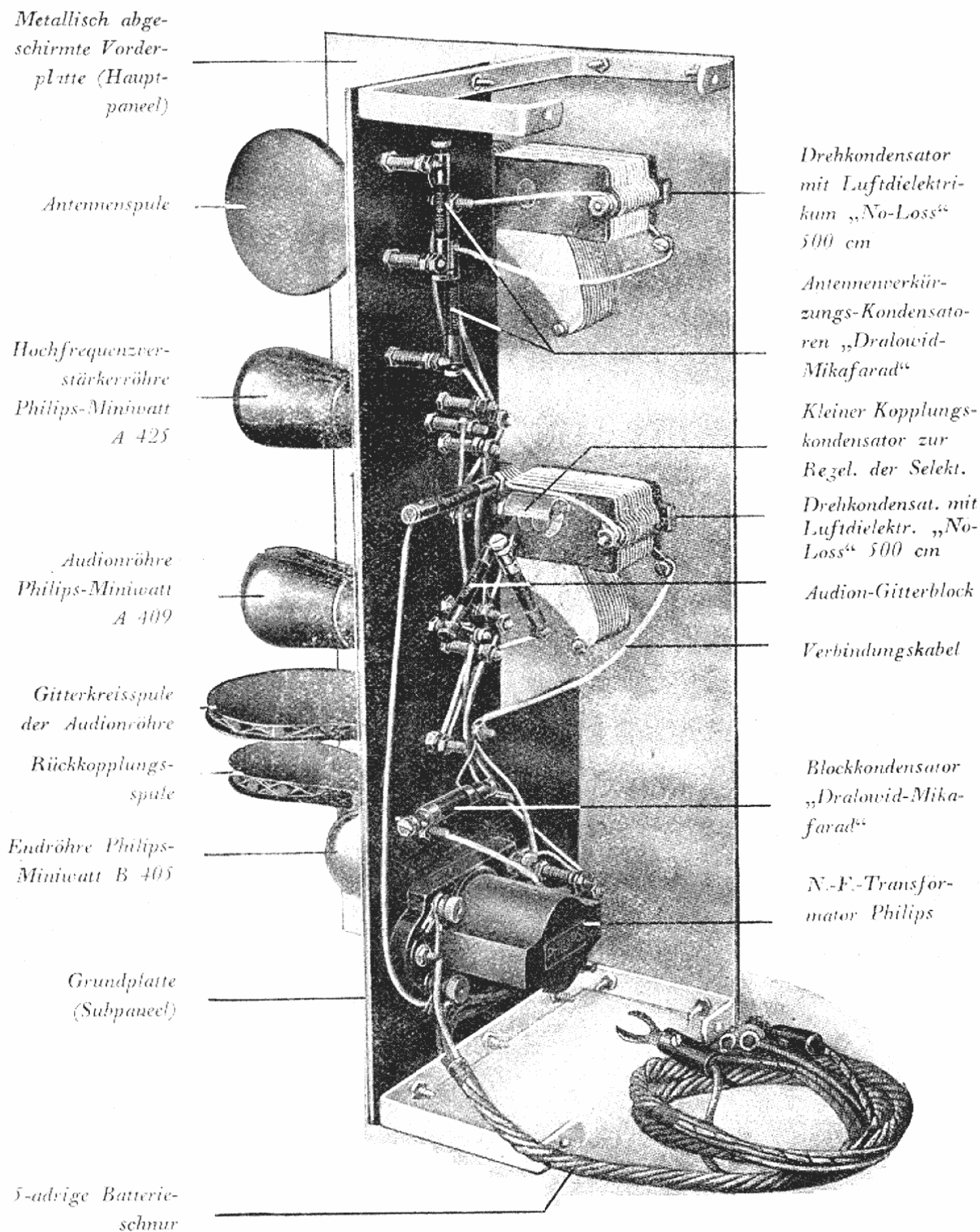
Ansicht des zusammengebauten Philips-Volks-empfangers von unten.
