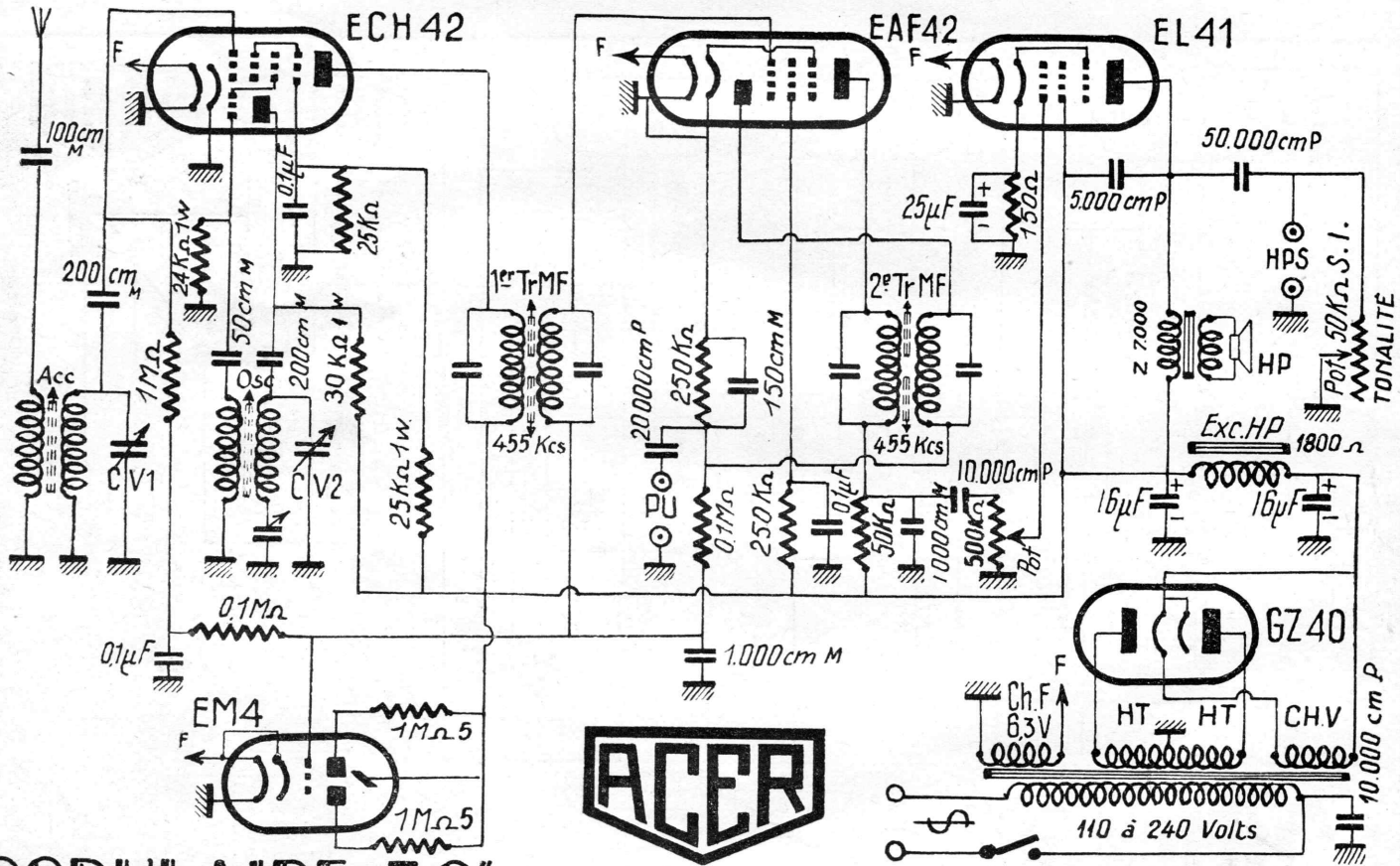
"POPULAIRE 50" 5 Lampes alternatif "RIMLOCK".
