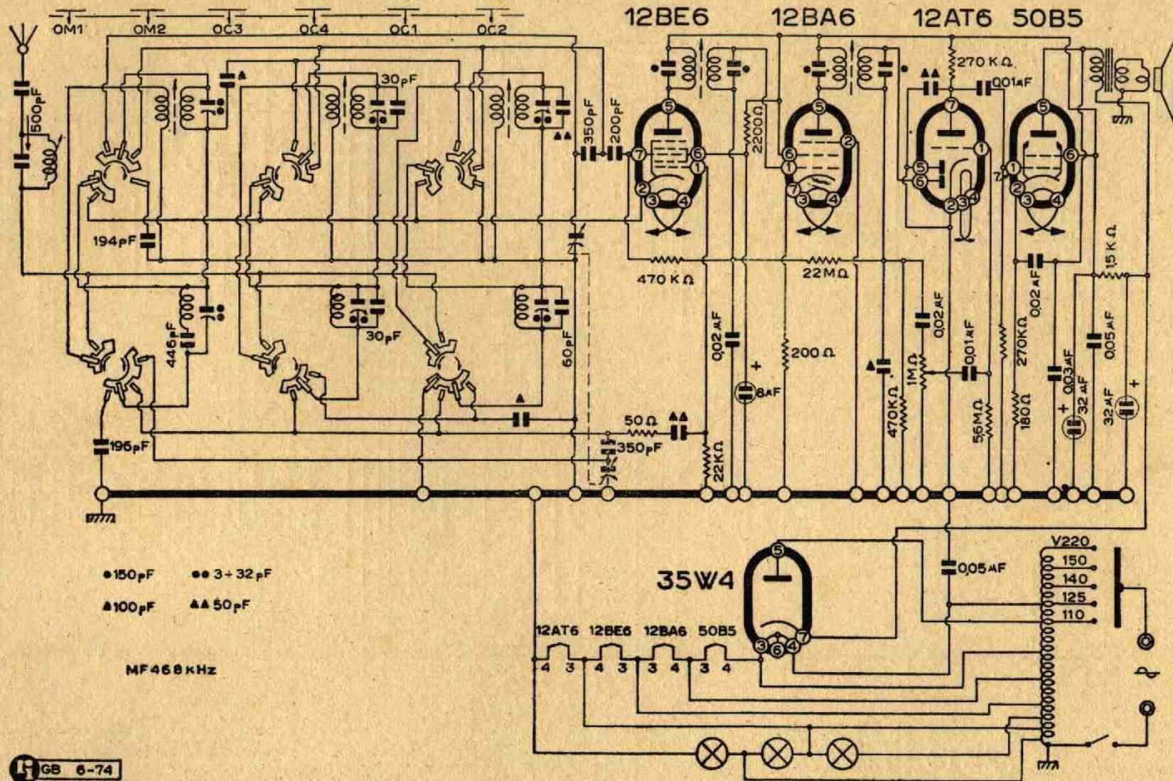
Lo schema elettrico del mod. Supergioiello c. a. 195
