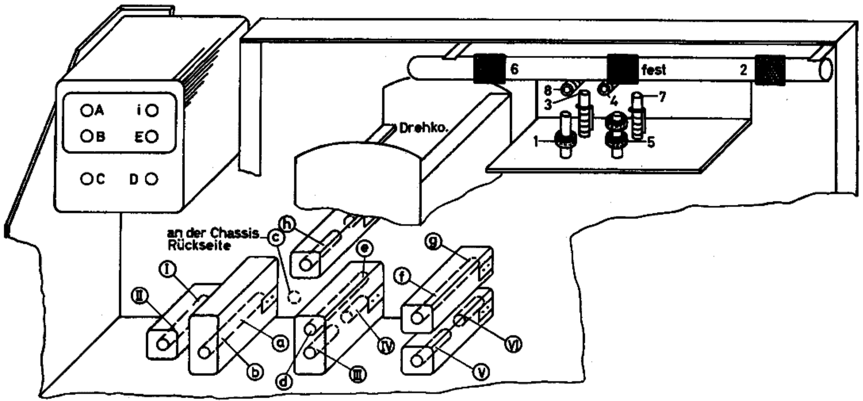
Abgleich-Lageplan
