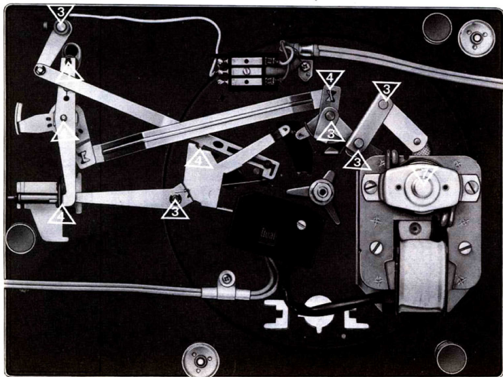
Fig. 10 Schmierstellen unter der Platine
