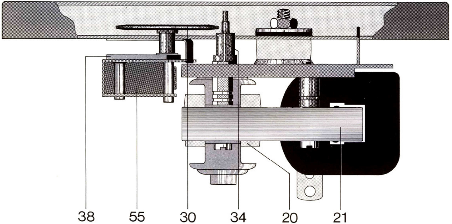
Fig. 1 Motoraufhängung und Antrieb des Plattentellers
