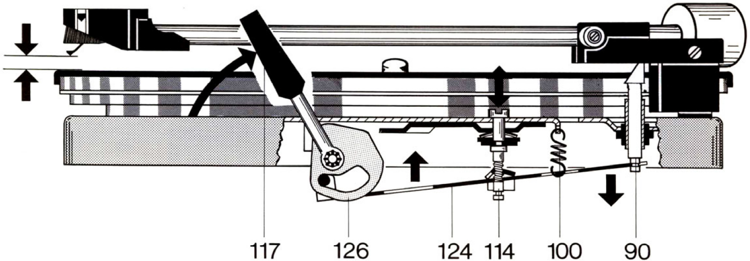
Fig. 4 Tonarmlift (Tonarm abgehoben).
