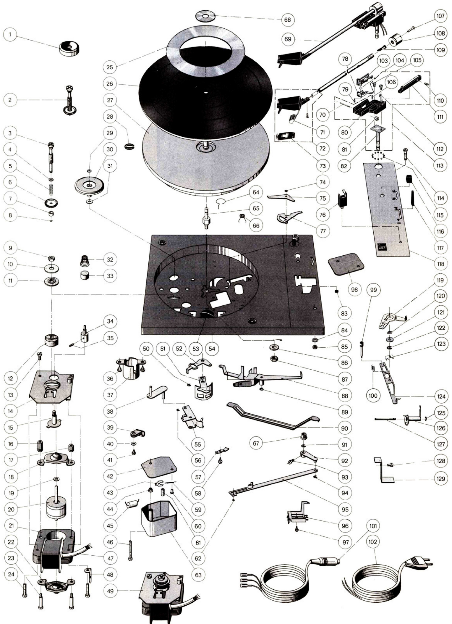
Fig. 11 Explosionsdarstellung
