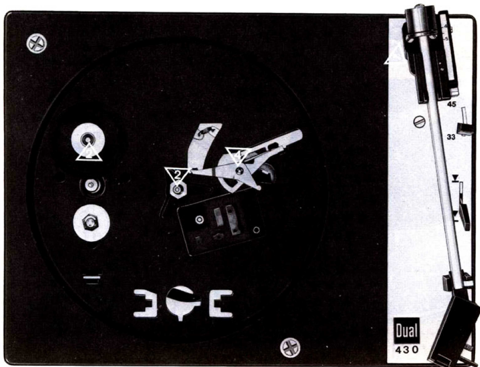
Fig. 9 Schmierstellen über der Platine
