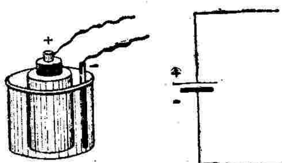
FIG. 25. — Comment on représente une pile sur un schéma. — P, élément de pile, représenté schématiquement à droite par deux traits, un trait long et fin pour le pôle positif, un trait gros et court pour le pôle négatif de cet élément.
