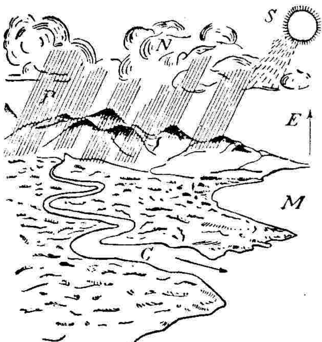
FIG. 29. — Représentation de la circulation de l'eau à la surface de la terre. — Elle est en tous points comparables à la circulation de l'électricité dans un réseau. L'eau de la mer M est évaporée par la chaleur du soleil S sous la forme de nuages N, qui accumulent la vapeur d'eau à de grandes hauteurs. Les nuages crèvent ensuite en donnant des précipitations de pluie, de neige ou de grêle sur des régions plus ou moins élevées, d'où cette eau ruisselle ensuite en rivières C vers la mer, en restituant toute l'énergie mécanique potentielle que le soleil lui avait communiquée dans son ascension nébuleuse.
