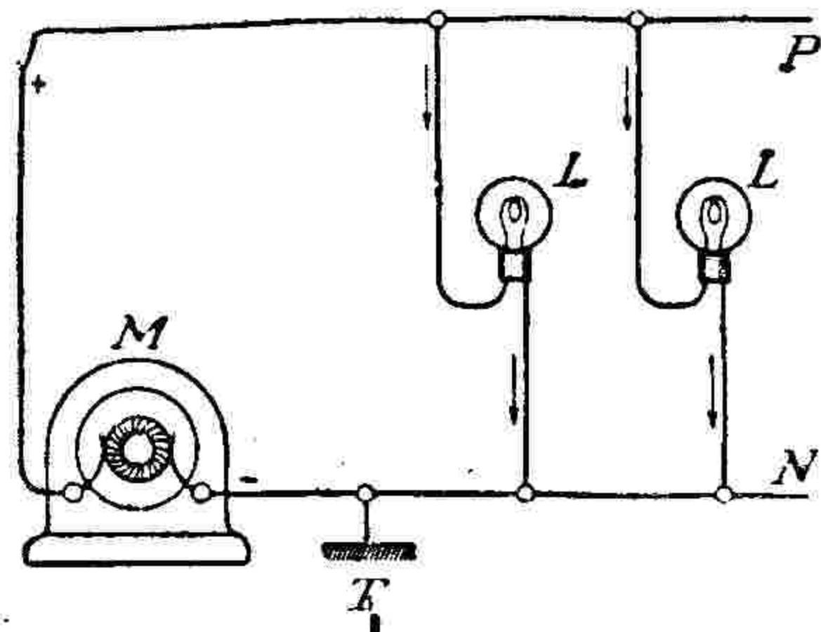
FIG. 27. — Représentation d'un réseau de courant électrique continu. — M, machine produisant à l'usine l'électricité qu'elle refoule d'une part dans le fil positif P, d'autre part dans le fil négatif N, qui peut être relié à la terre T. Les appareils d'utilisation, les lampes L, par exemple, sont branchées entre le fil positif et le fil négatif du réseau. Les flèches indiquent le sens des courants qui les parcourent.
