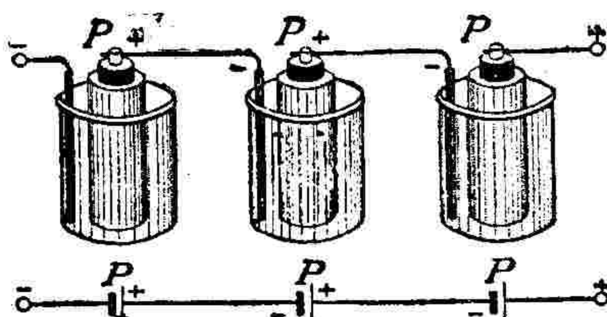
FIG. 26. — Représentation d'une batterie de piles. — La batterie de piles est obtenue en réunissant en « série » un certain nombre d'éléments de pile P, en reliant ensemble par un fil métallique le pôle positif de l'une et le pôle négatif de la suivante.
