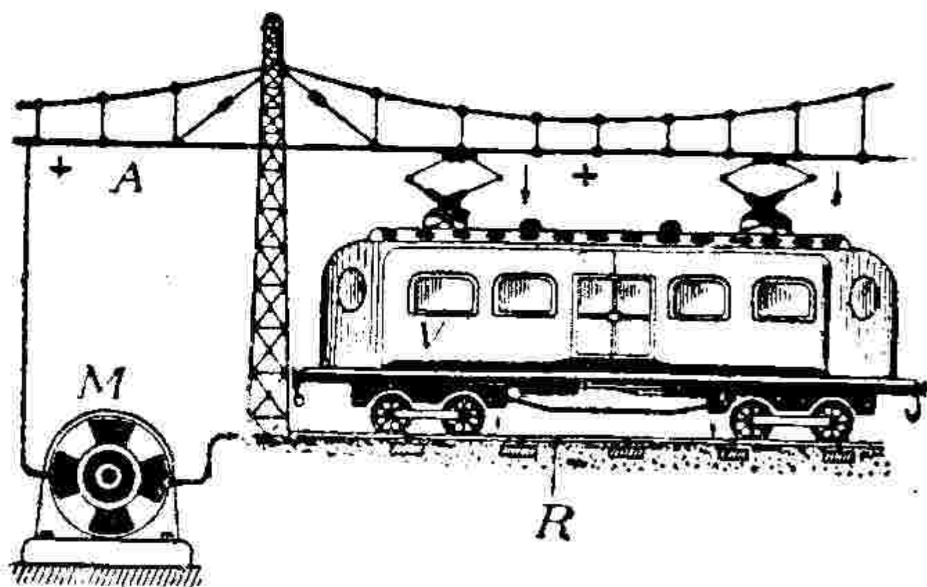
FIG. 28. — Représentation d'un réseau de traction à courant continu. — La tension électrique produite à l'usine par la machine M est envoyée par le pôle positif à la ligne aérienne caténaire A, tandis que le pôle négatif est relié à la terre par les rails R de la voie. Le courant traverse les machines de la voiture motrice V en allant du fil A à la voie R, par laquelle il se referme vers la machine M.
