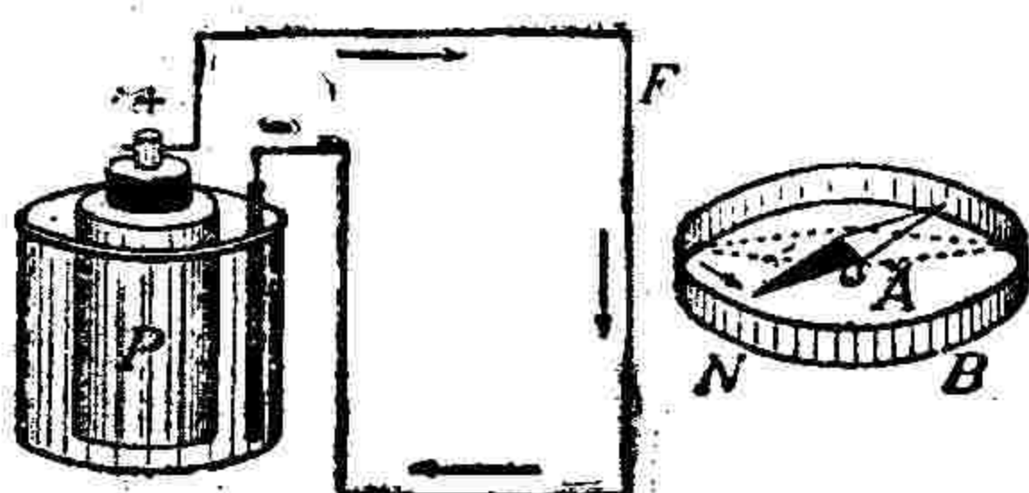
FIG. 24. — Comment reconnaître le sens d'un courant au moyen d'une boussole. — P, pile produisant le courant ; F, fil conducteur ; B, boussole ; A, aiguille aimantée ; N, pôle nord qui dévie à gauche sous l'action d'un courant vertical.
