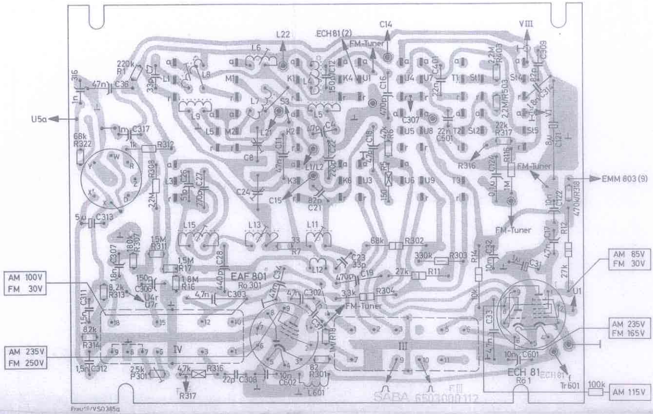
HF-Platte
