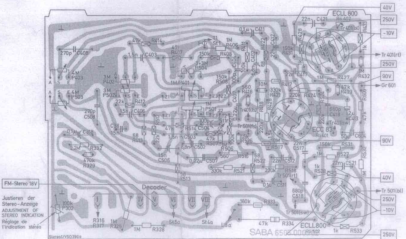
NF-Platte
