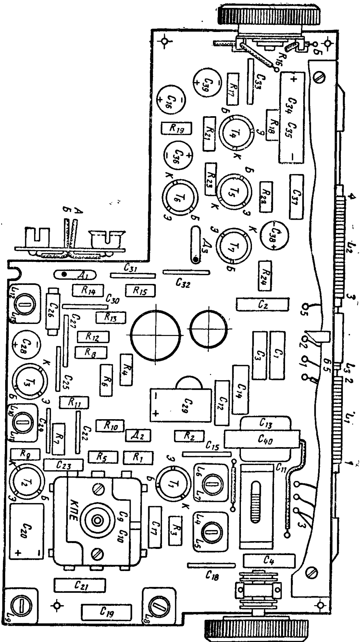
Рис. 4.30. Схема расположения узлов и деталей на печатной плате приемника «Этюд».
