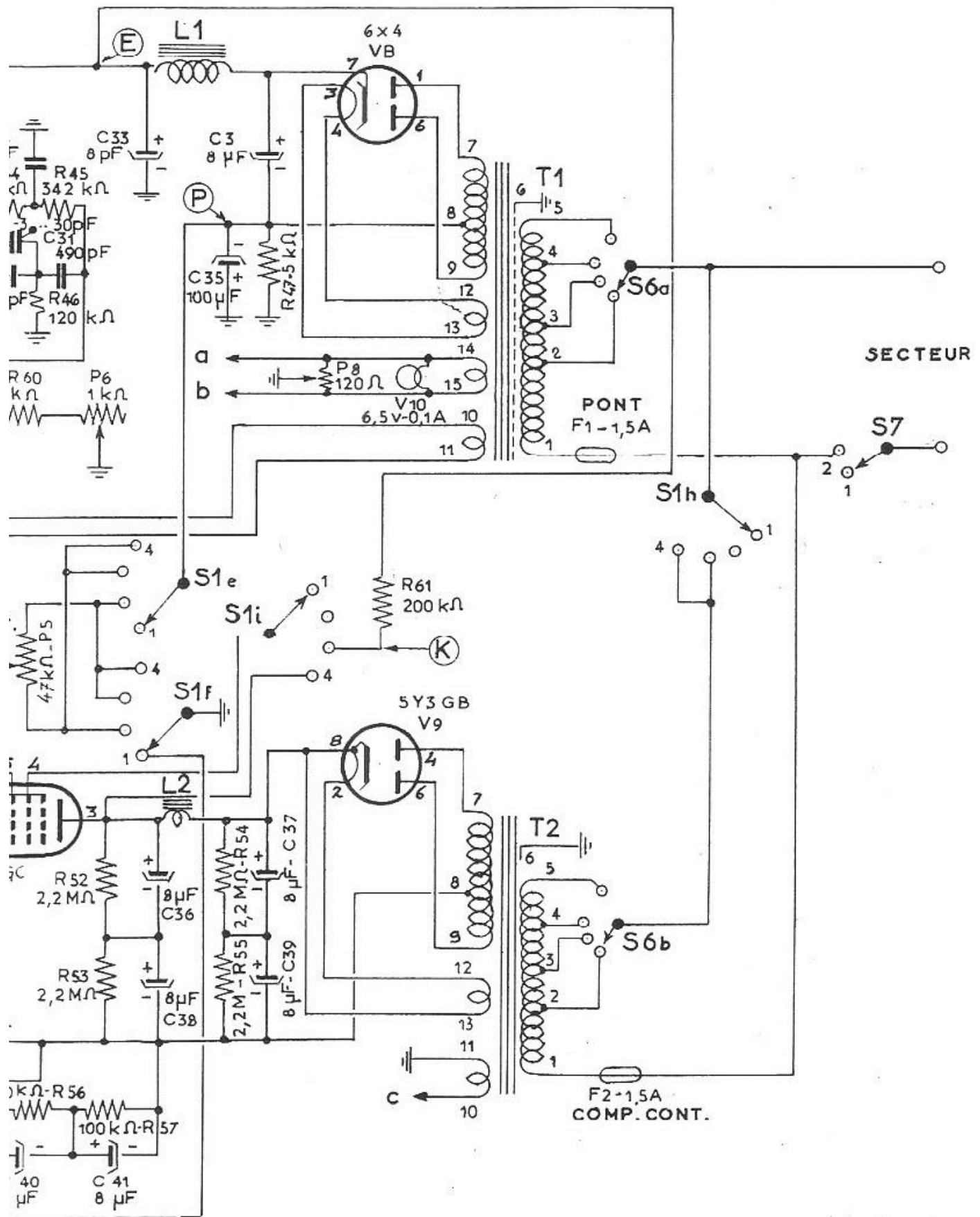
PONT D'IMPÉDANCES 626 B MÉTRIX. SCHEMA DE PRINCIPE
