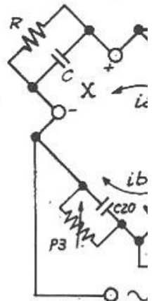
Mesure des capacités
