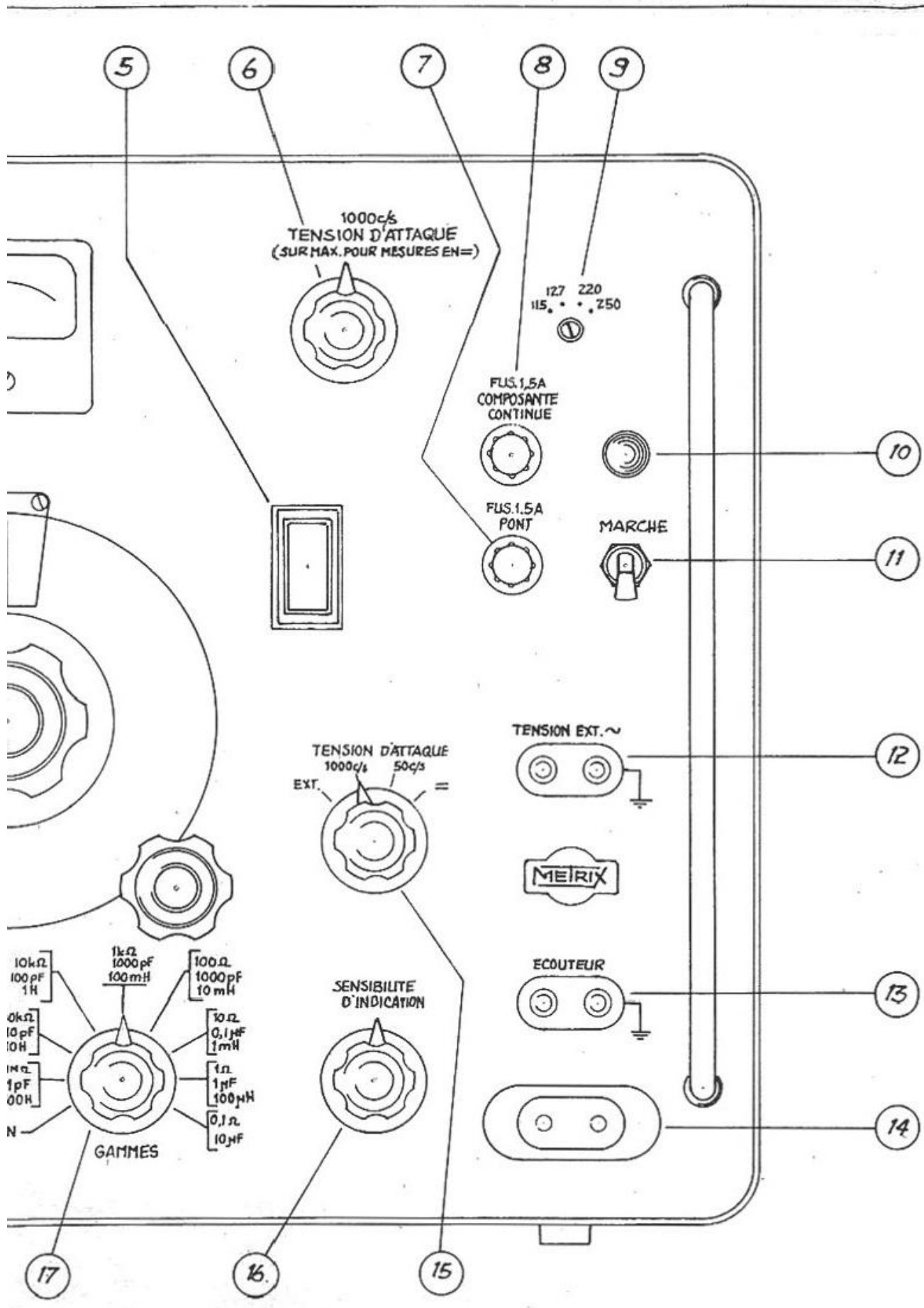
VUE AVANT DU PONT 626 B_METRIX_
