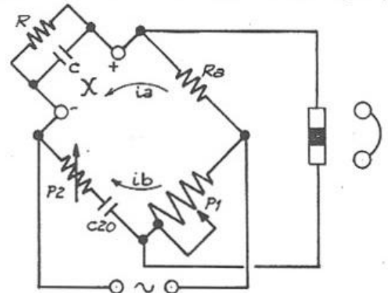
Mesure des capacités à faible perte \text{tg } \delta < 0,1
