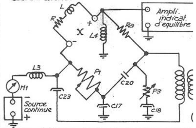
Mesure des capacités à faible perte \text{tg } \delta < 0,1
