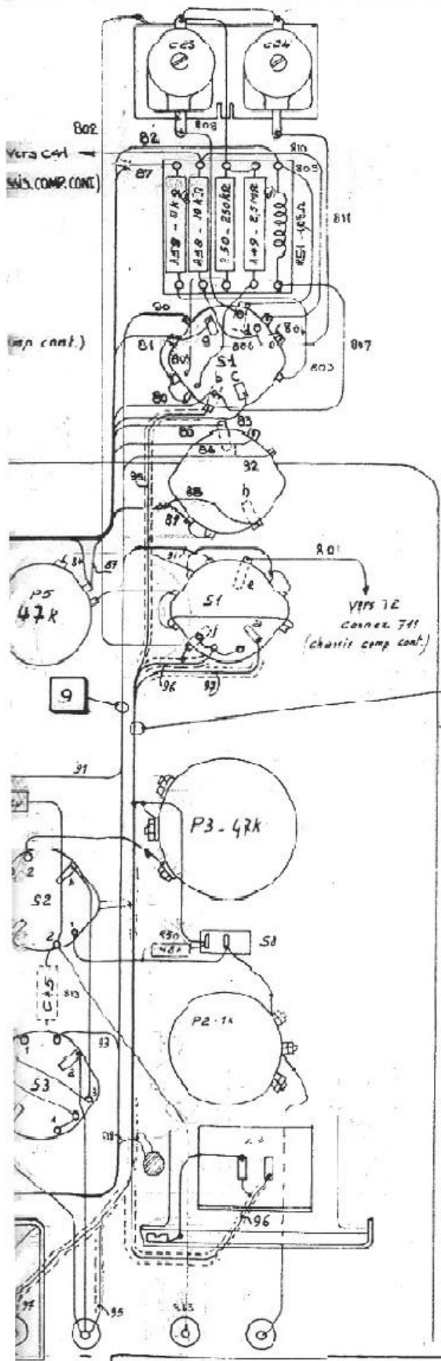
PONT D'IMPÉDANCES 626B METRIX
