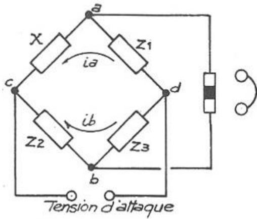
Mesure des résistances
