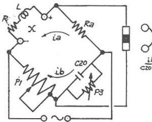
Mesure des inductances à faible surtension Q < 10
