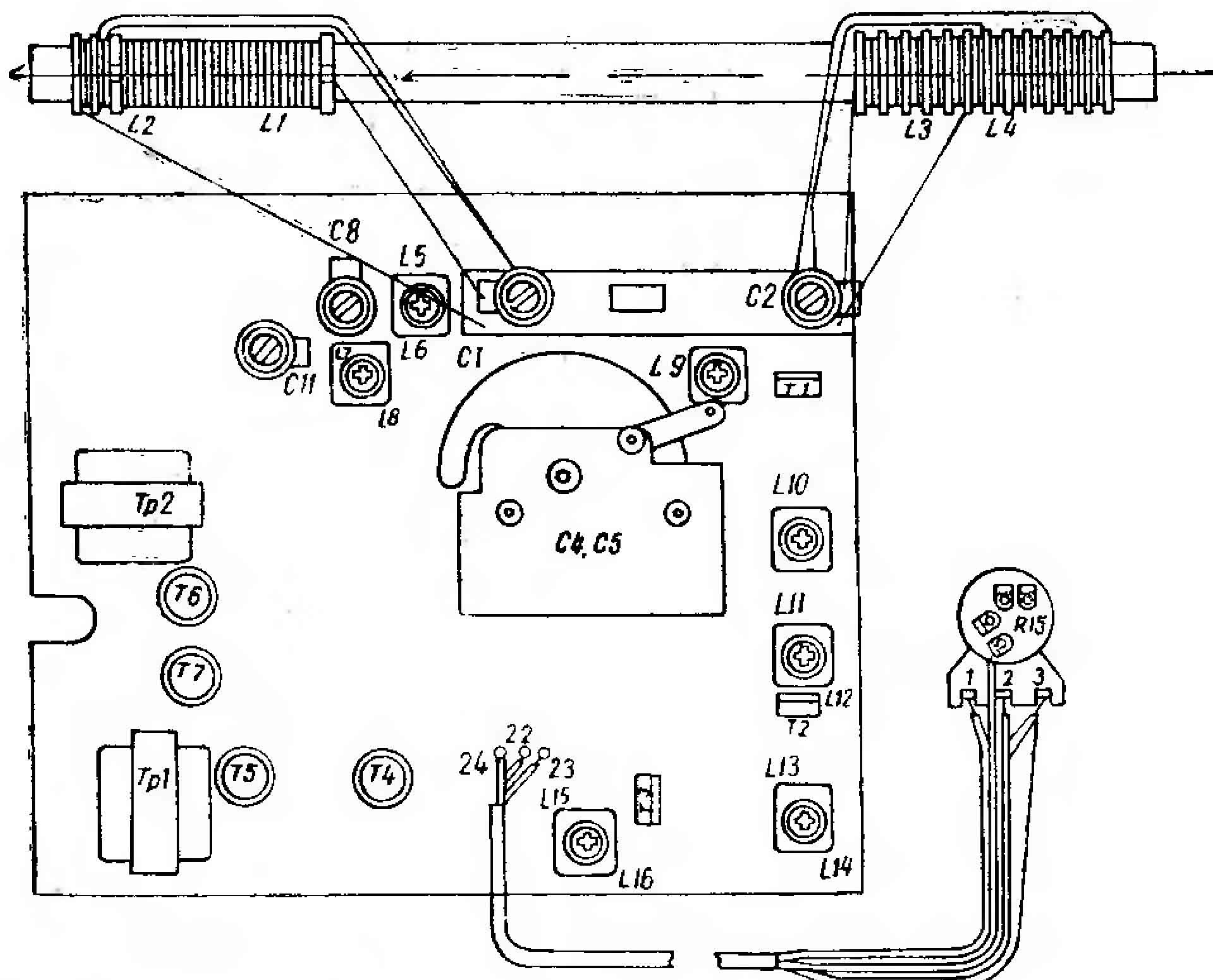
Вид платы сверху с расположением основных узлов
