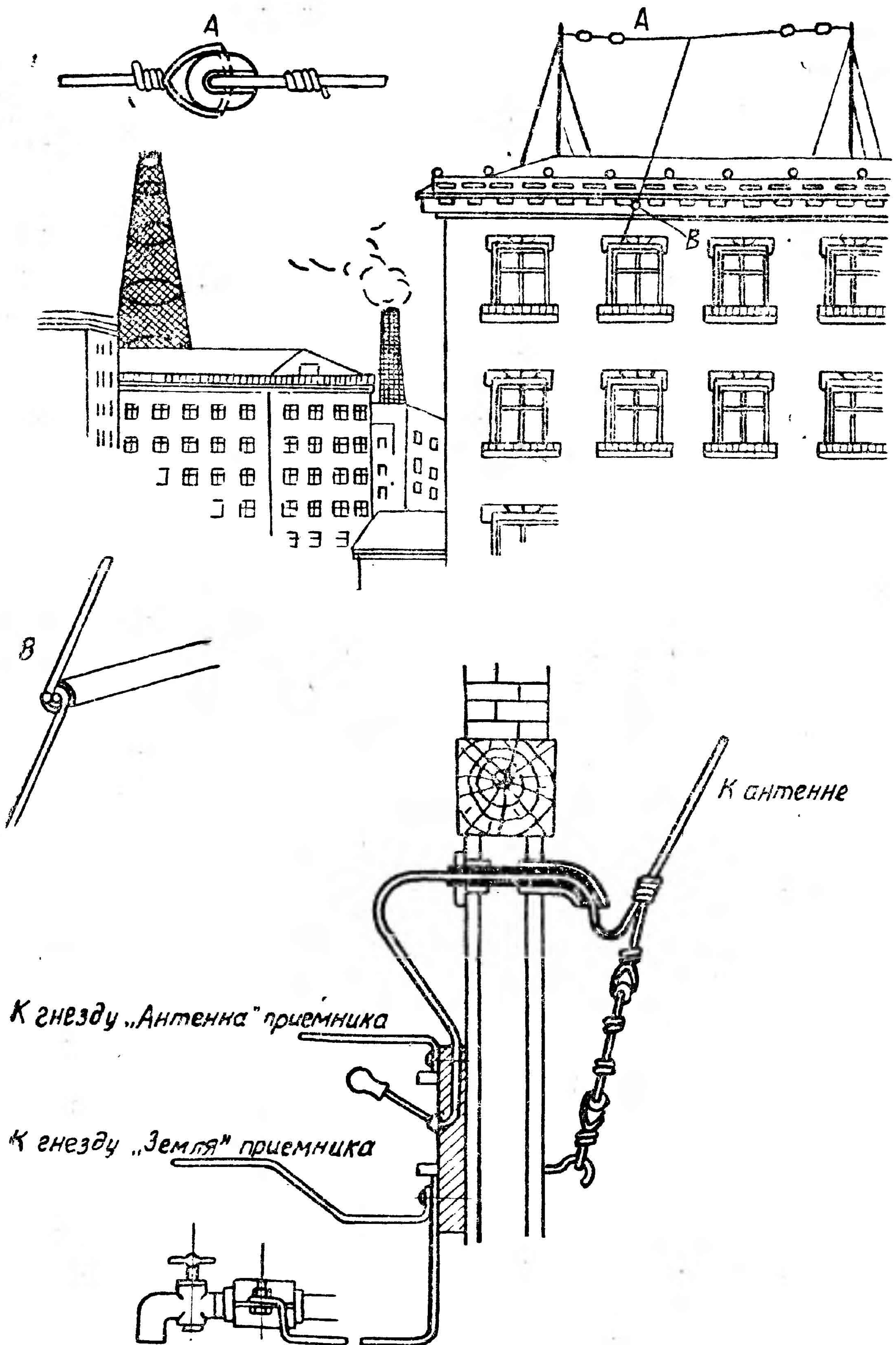
Рис. 3. Устройство антенны
