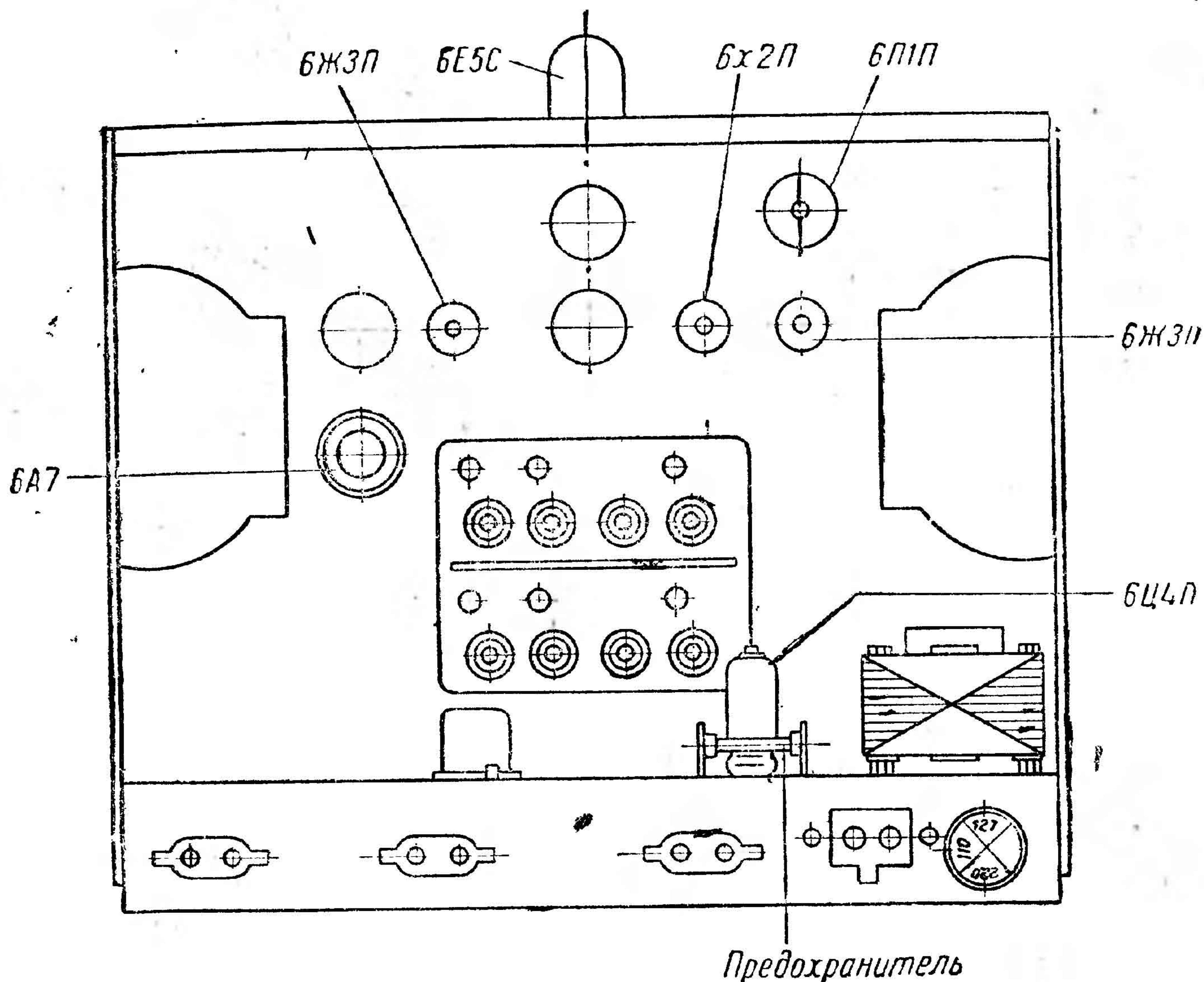
Рис. 2. Расположение ламп на шасси
