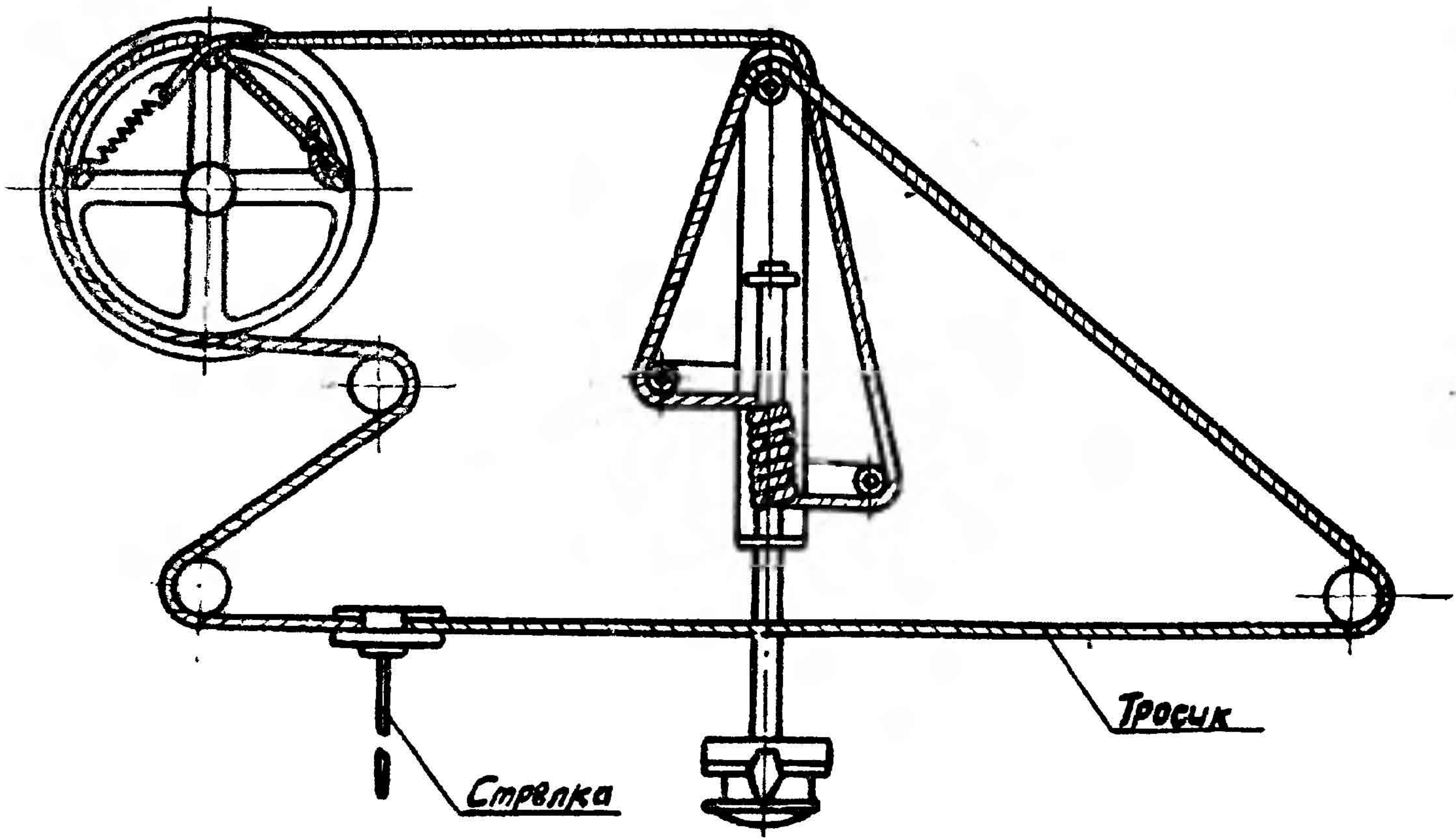
Рис. 4. Схема верньерного устройства приемника Звезда-54
