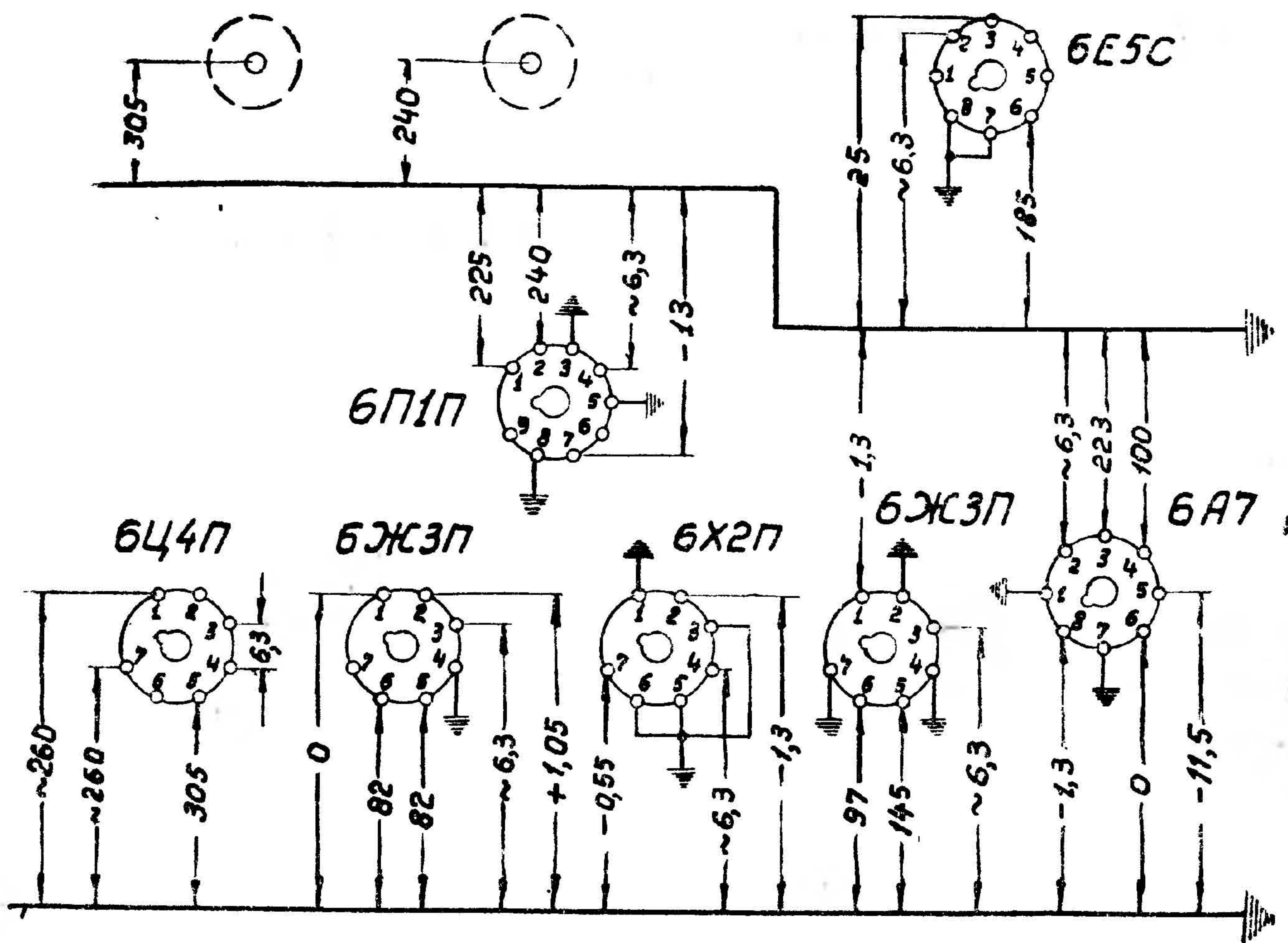
Диаграмма напряжений приемника „Звезда-54”
