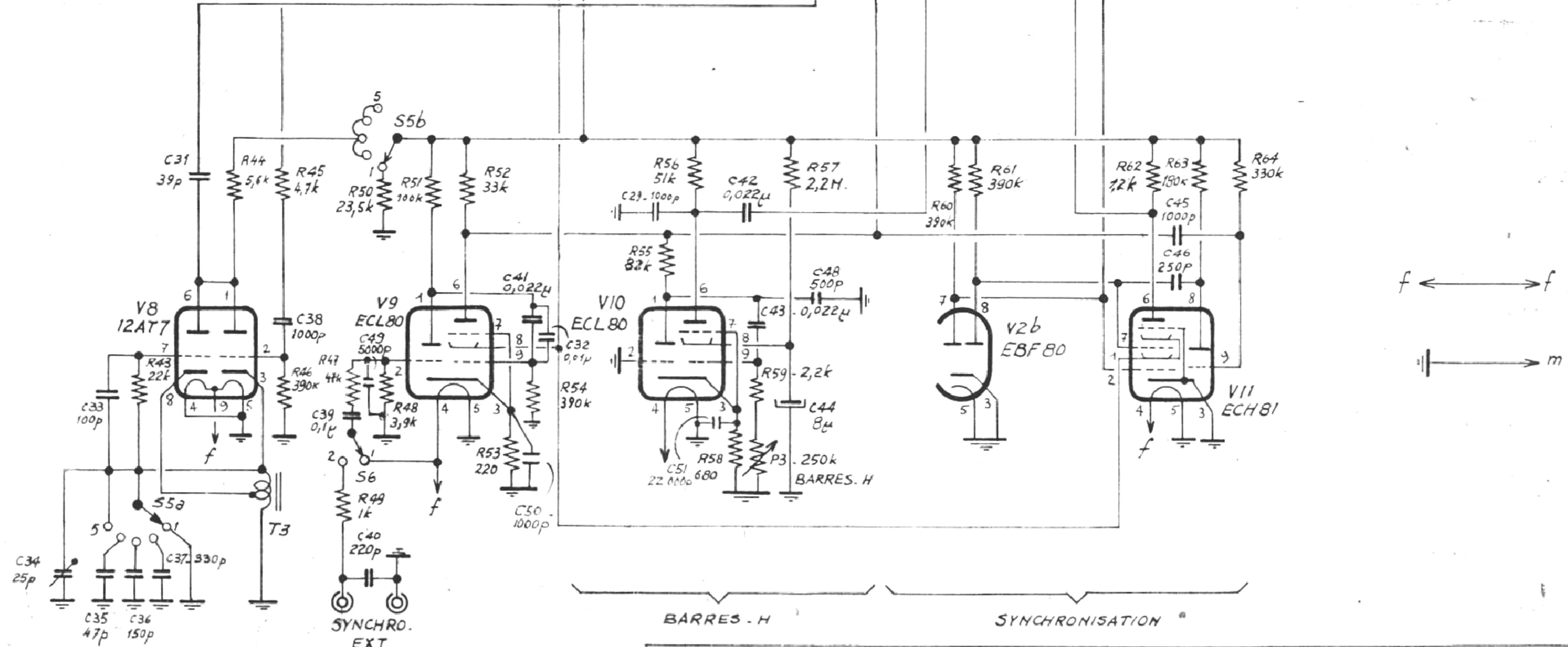
SCHEMA DE PRINCIPLE MIRE 265 METRIX - PARTIE VIDEO -
