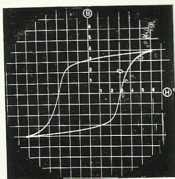
COURBE D'HYSTERESIS DE LA BANDE WSM
