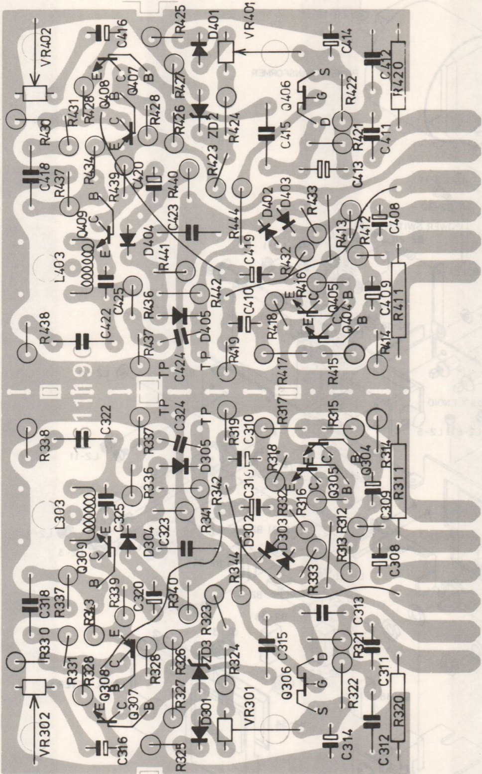
Dolby - Leiterplatte
