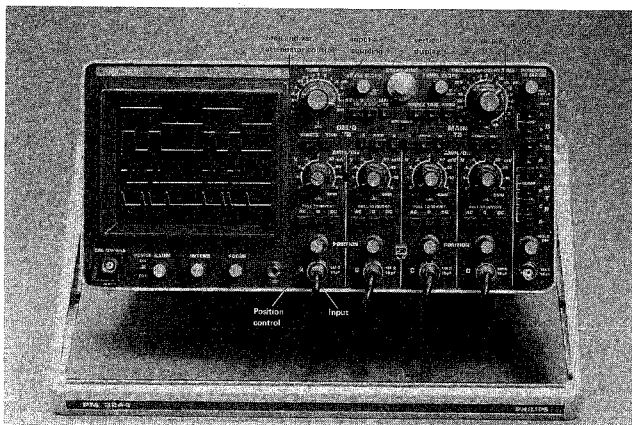
Abb. 2.3. Vertikalablenkung
