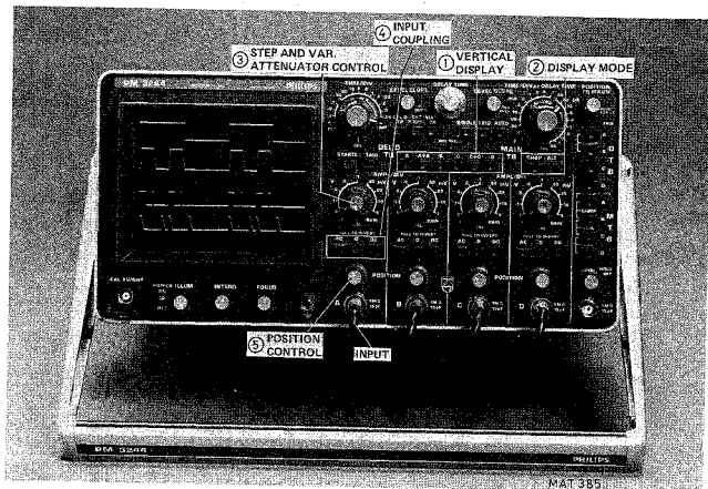
Abb. 2.3. Vertikalablenkung
