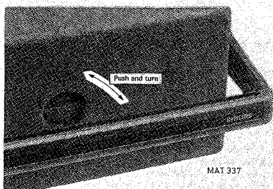
Fig. 2.1. Dépose du couvercle frontal
