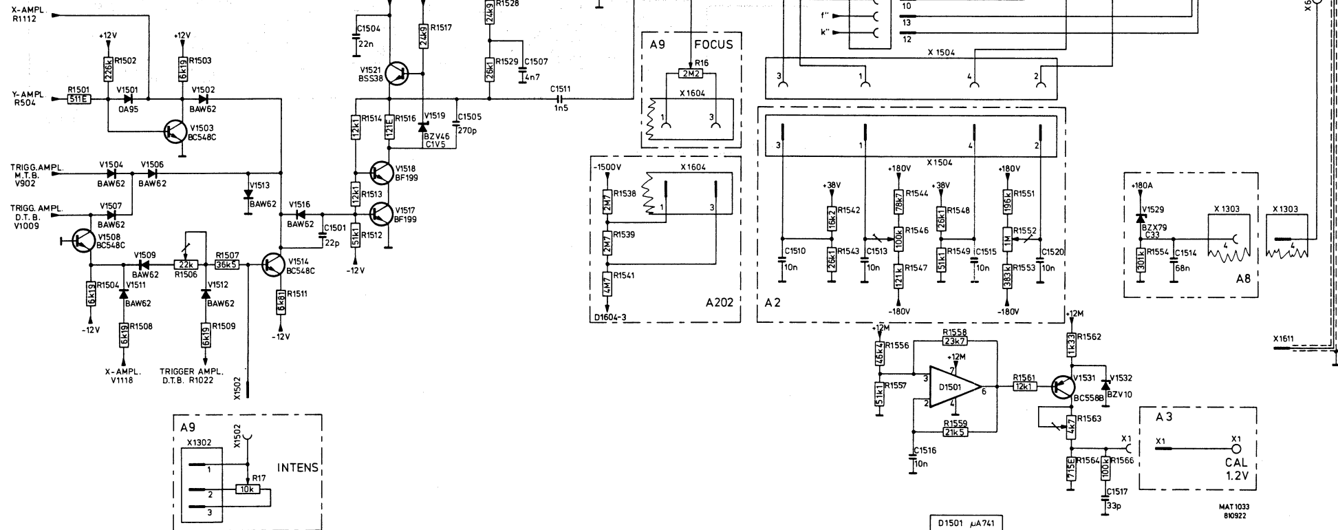
Fig. 8.8. Z-Amplifier
