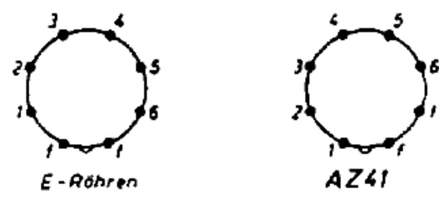
Sockelschaltung
